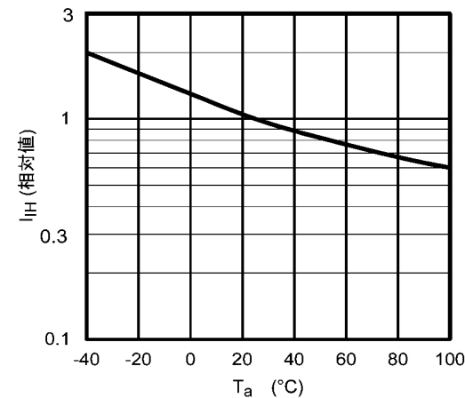
图 12.11 相对 I_H - T_a
