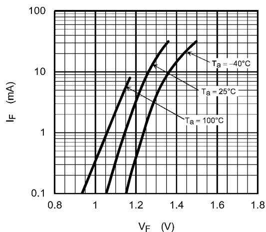
図 12.3 I_F - V_F
