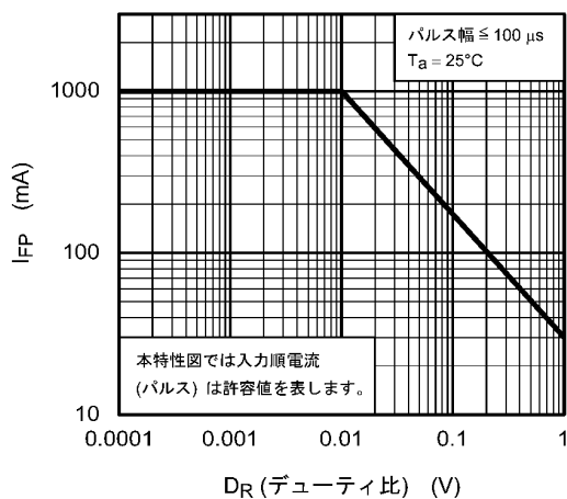
図 12.4 I_{FP} - D_R
