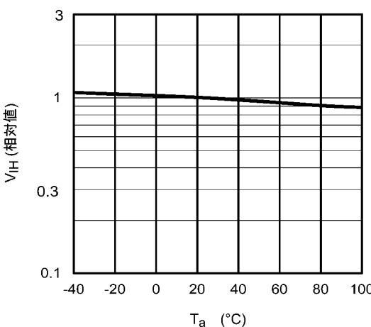
图 12.10 相对 V_H - T_a
