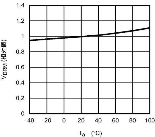
图 12.8 相对 V_{DRM} - T_a
