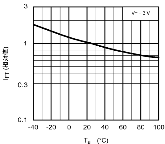
図 12.6 相対 I_{FT} - T_a
