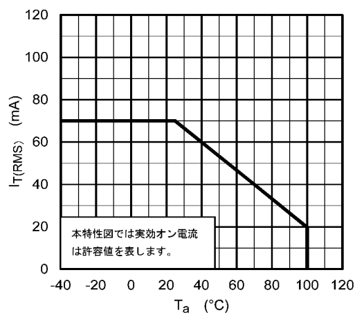
図 12.2 I_T(RMS) - T_a
