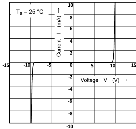
図 8.1 I - V
