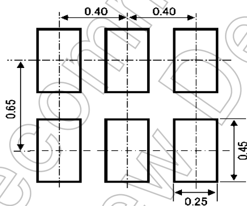
図 7.1 参考パッド寸法 (Unit: mm)
