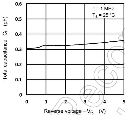
図 8.3 C_t - V_R
