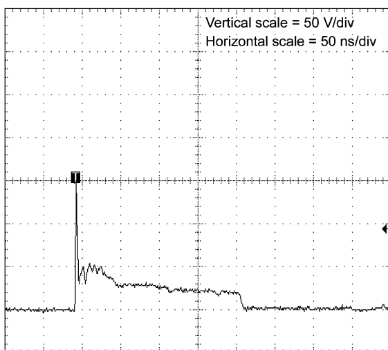
図 11.1 +8 kV
