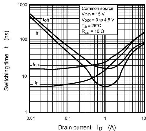
Fig. 8.11 t - I_D
