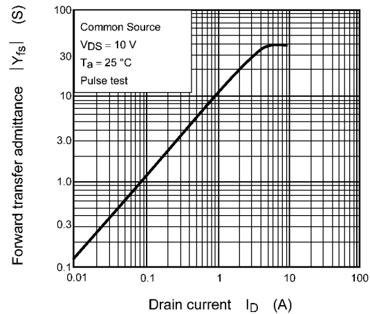
Fig. 8.8 |Y_{fs}| - I_D
