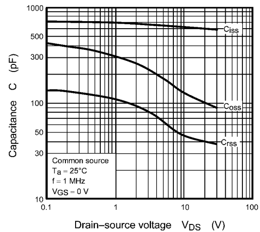
Fig. 8.10 C - V_{DS}
