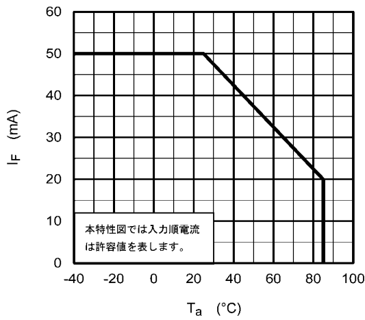
図 12.1.1 I_F - T_a
