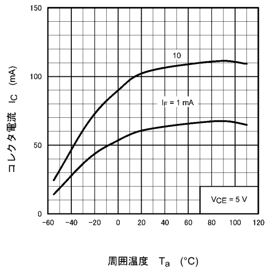
図 11.12 I_C - T_a
