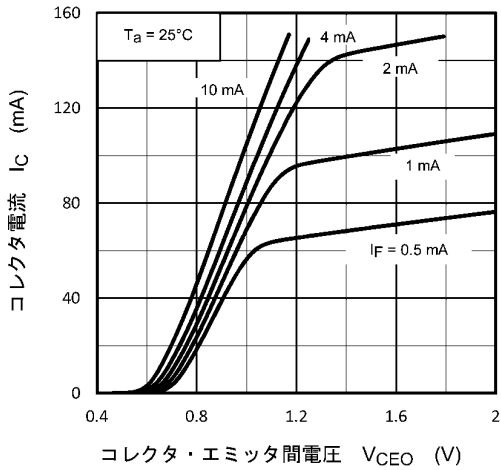
図 11.7 I_C - V_{CE0}
