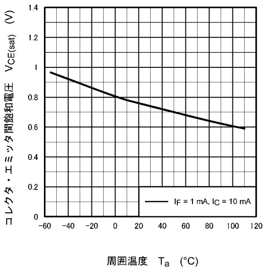
図 11.11 V_{CE(sat)} - T_a
