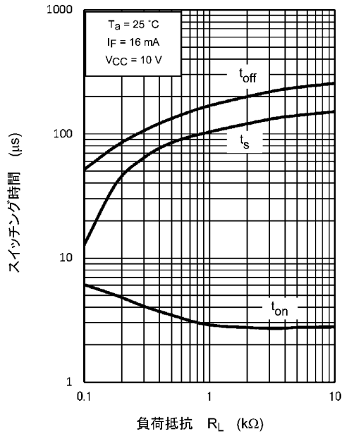
図 11.13 スイッチング時間 - R_L
