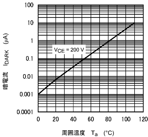
図 11.9 I_{DARK} - T_a
