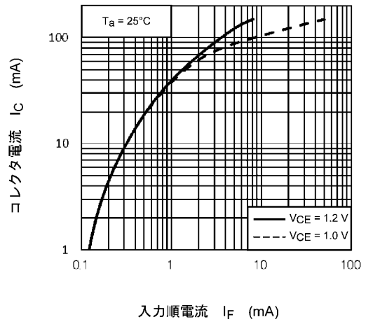
図 11.8 I_C - I_F
