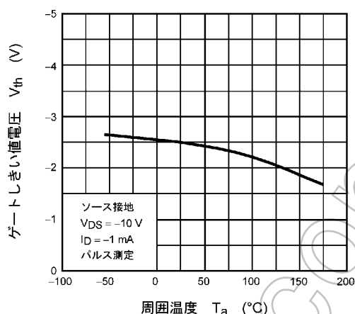
図 8.9 V_{th} - T_a (注8)
