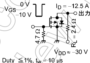
図 6.2.1 スwitchング時間の測定回路例
