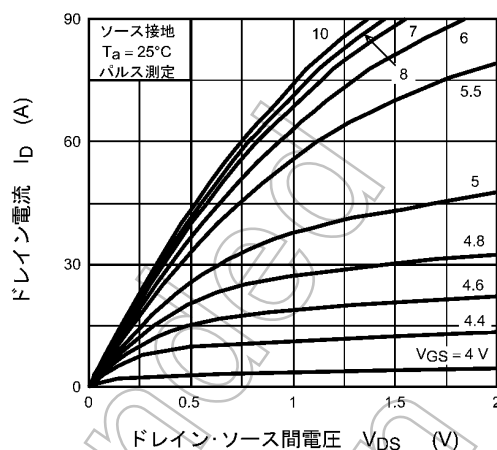
図 8.2 I_D - V_{DS}
