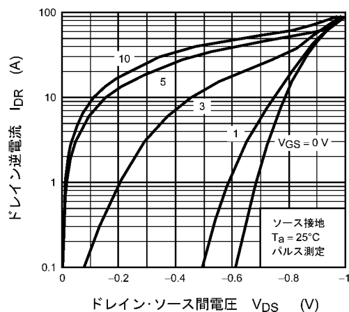
図 8.7 I_{DR} - V_{DS}
