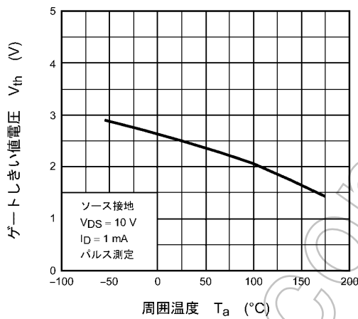
図 8.9 V_{th} - T_a (注7)
