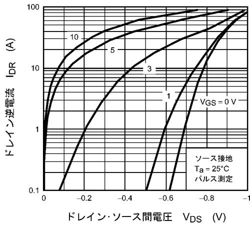
図 8.7 I_{DR} - V_{DS}
