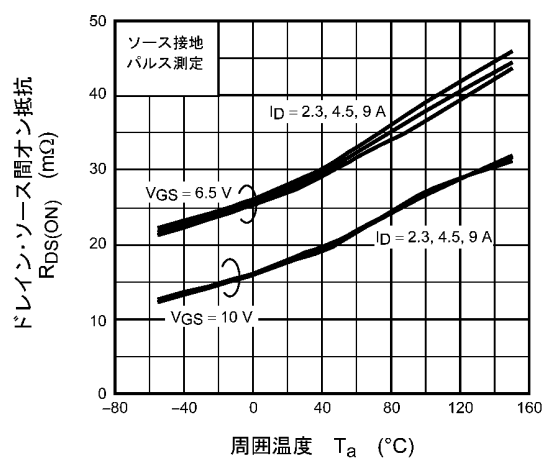
図 8.6 R_{DS(ON)} - T_a
