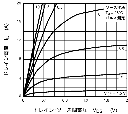
図 8.2 I_D - V_{DS}
