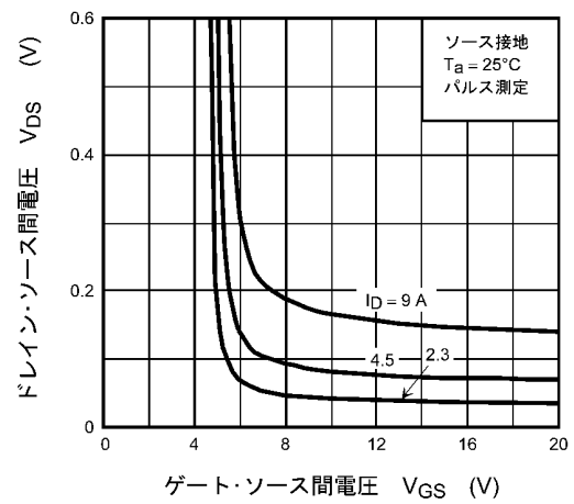
図 8.4 V_{DS} - V_{GS}
