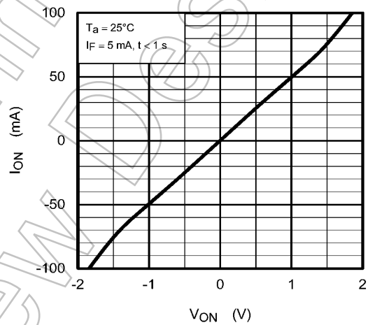
図 13.1.4 I_{ON} - V_{ON}
