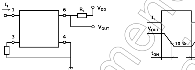
図 12.1 スイッチング時間測定回路, 波形
