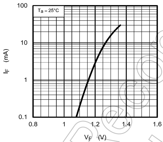
図 13.1.3 I_F - V_F
