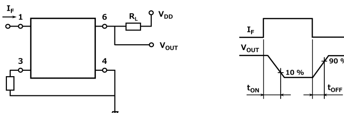
図 12.1 スイッチング時間測定回路, 波形
