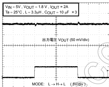
モード切替 I_{OUT} = 2A (パルススキップ→連続 PWM→パルススキップ)
