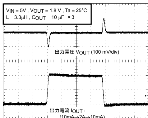
負荷応答特性 (連続 PWM モード)
