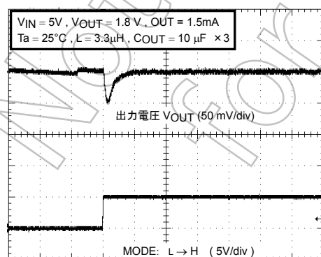
モード切替 I_{OUT} = 1.5mA (パルススキップ→連続 PWM)
