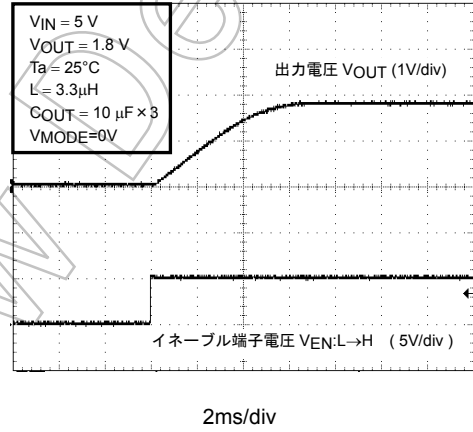
起動特性 (パルススキップ付きモード ソフトスタート時間)
