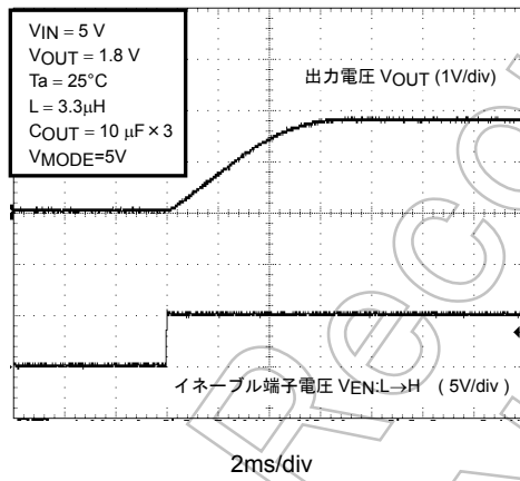
起動特性 (連続 PWM モード ソフトスタート時間)
