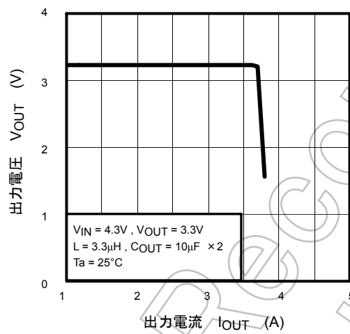
過電流特性
