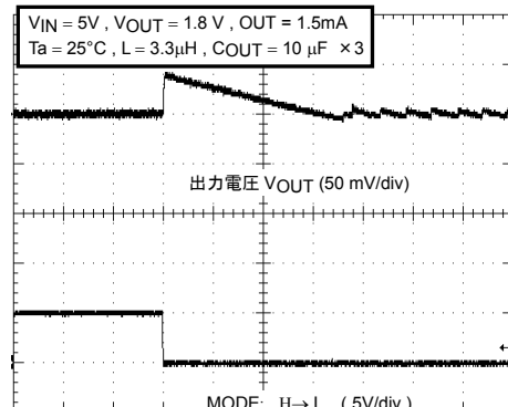
モード切替 I_{OUT} = 1.5mA (連続 PWM→パルススキップ)
