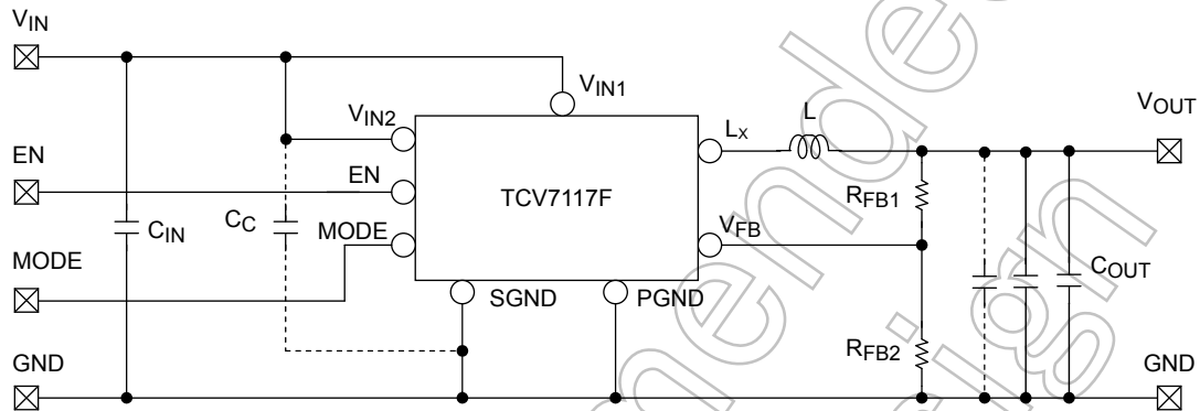
図 1 TCV7117F 応用回路例
