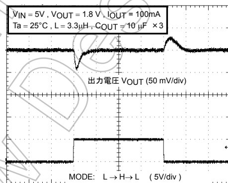
モード切替 I_{OUT} = 100mA (パルススキップ→連続 PWM→パルススキップ)
