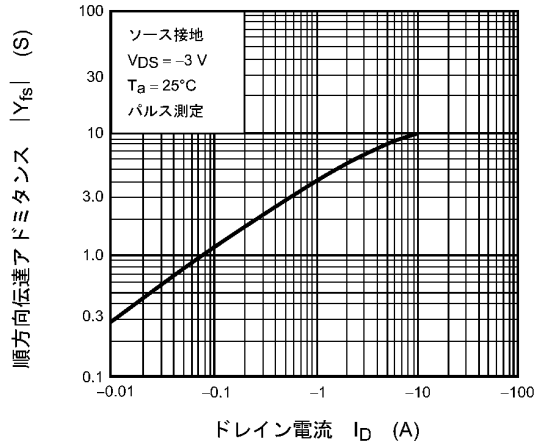
図 7.8 |Y_{fs}| - I_D
