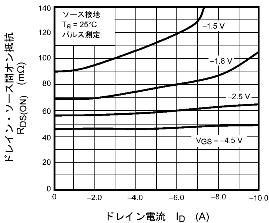
図 7.5 R_{DS(ON)} - I_D
