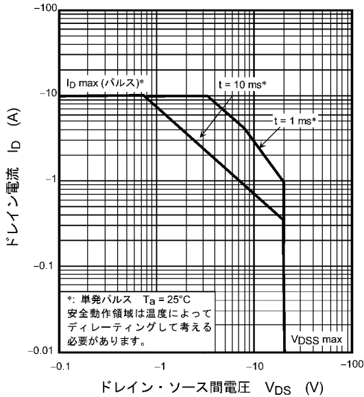
図 7.15 安全動作領域
