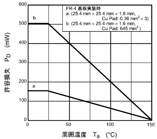
図 7.12 P_D - T_a
