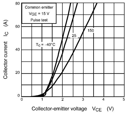
Fig. 8.4 I_C - V_{CE}
