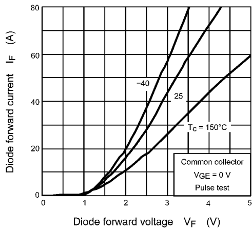
Fig. 8.12 I_F - V_F
