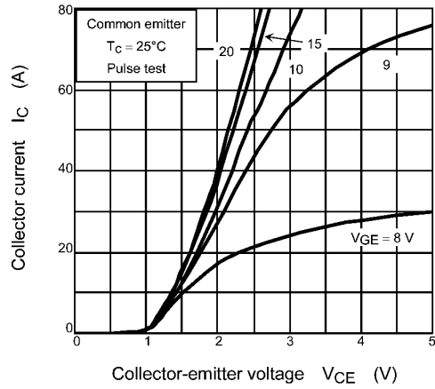
Fig. 8.2 I_C - V_{CE}
