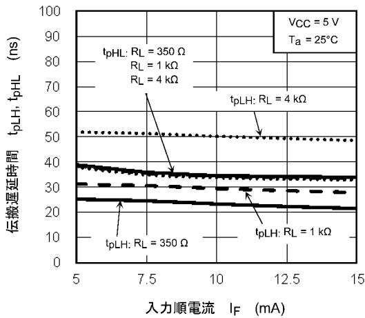
図 13.2.15 t_{pLH} / t_{pHL} - I_F
