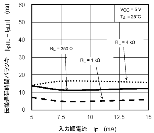
図 13.2.16 |t_{pHL} - t_{pLH}| - I_F
