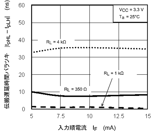
図 13.2.18 |t_{pHL} - t_{pLH}| - I_F
