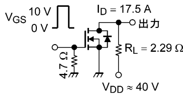
図 6.2.1 スwitching時間の測定回路例
