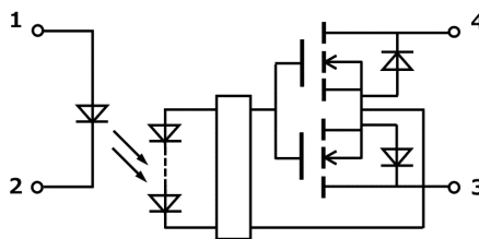
図 5.1 内部回路構成
