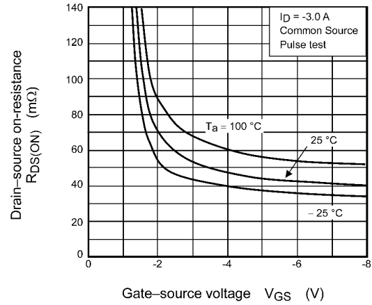
Fig. 8.4 R_{DS(ON)} - V_{GS}
