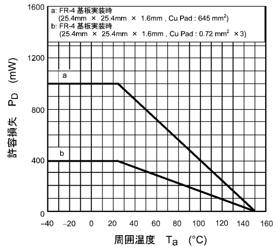
図 9.14 P_D - T_a
