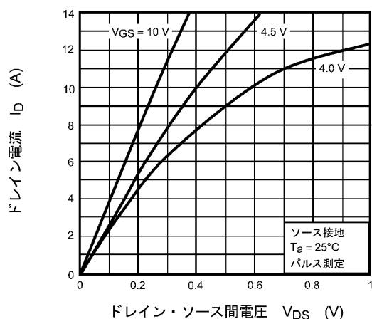
図 9.1 I_D - V_{DS}
