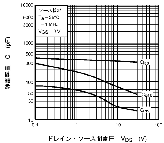
図 9.10 C - V_{DS}
