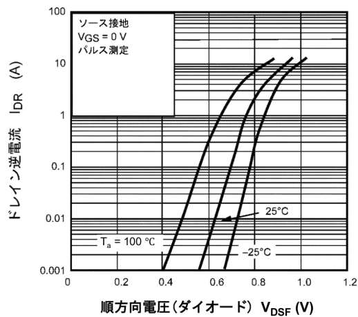
図 9.9 I_{DR} - V_{DSF}
