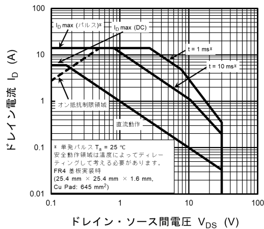
図 9.15 安全動作領域
