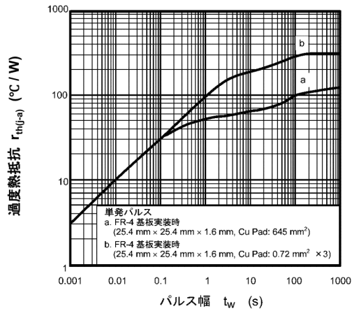
図 9.13 r_{th(j-a)} - t_w
