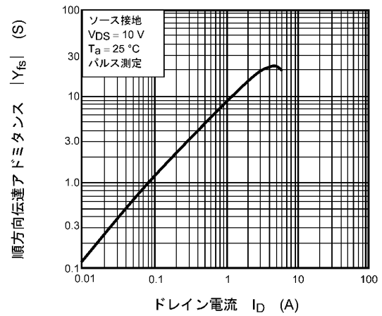
図 9.8 |Y_{fs}| - I_D
