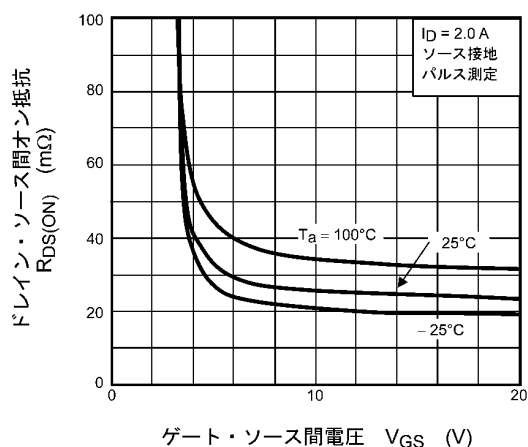
図 9.3 R_{DS(ON)} - V_{GS}
