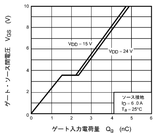
図 9.12 ダイナミック入力特性
