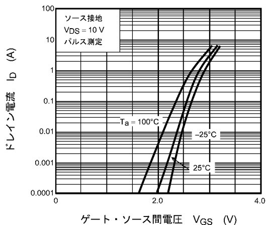
図 9.2 I_D - V_{GS}
