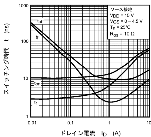
図 9.11 t - I_D
