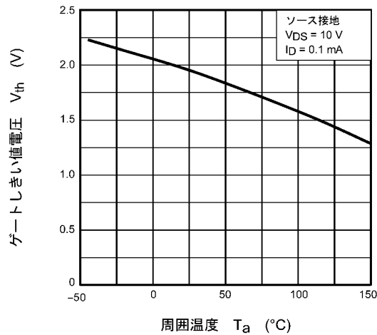
図 9.7 V_{th} - T_a
