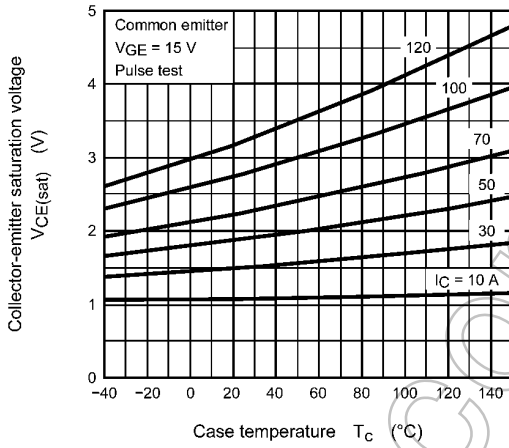
Fig. 8.9 V_{CE(sat)} - T_c
