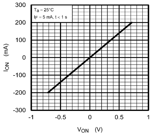
図 12.1.4 I_{ON} - V_{ON}
