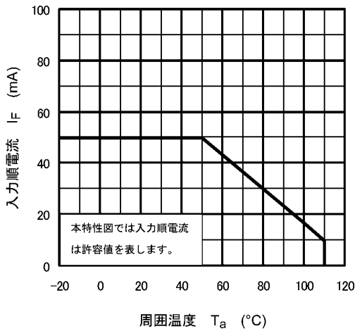
図 11.1 I_F - T_a
