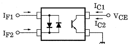
図 8.1 コレクタ電流比測定回路
