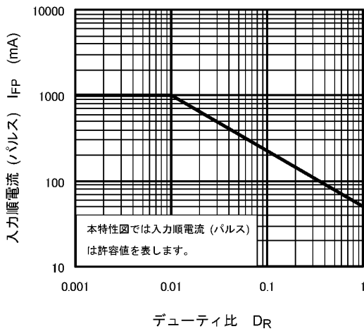
図 11.3 I_{FP} - D_R
