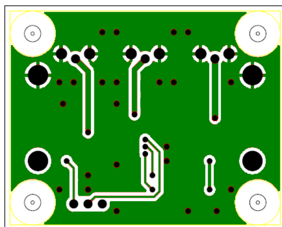
Bottom Layer
