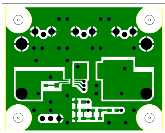
Top Layer
