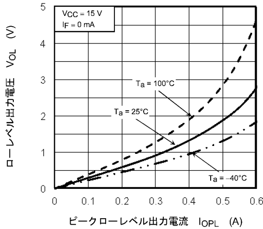
図 13.2.9 V_{OL} - I_{OPL}
