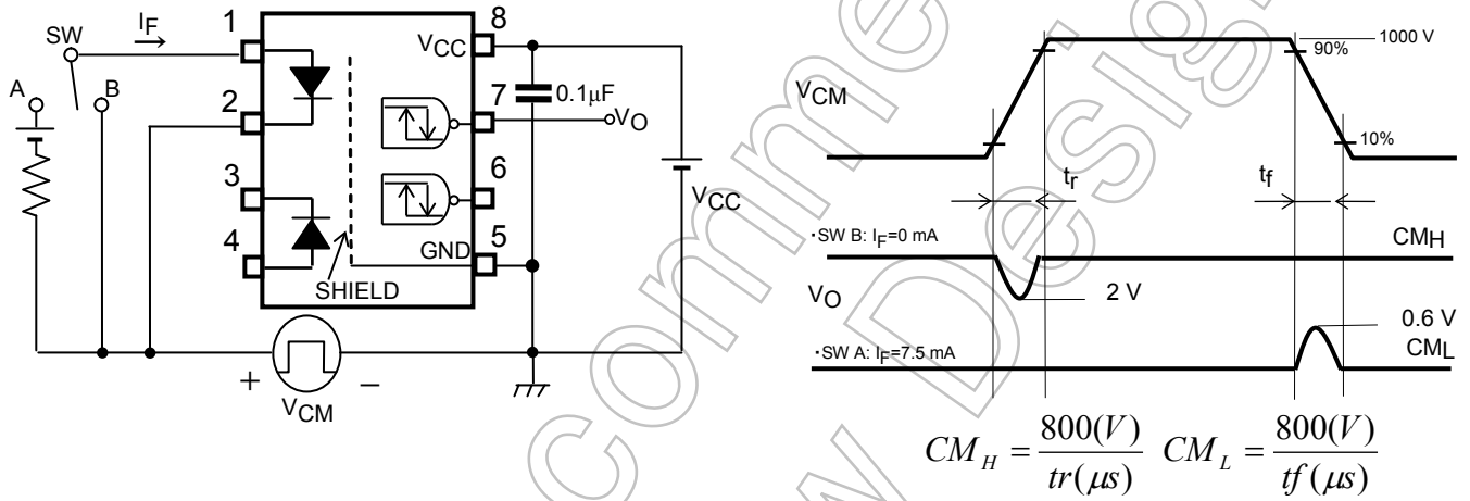
図 6: コモンモードノイズ除去電圧測定回路、波形
