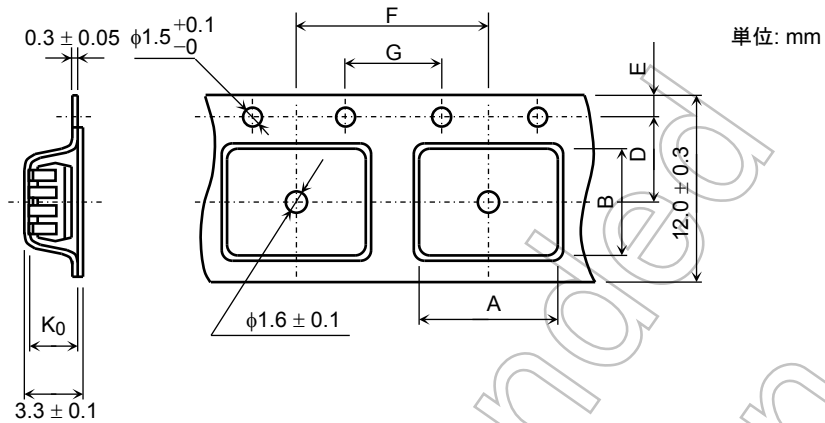
図 2 テーピング形状
