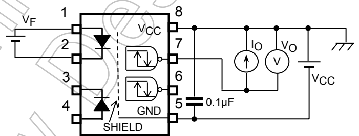
図 2: VOH 測定回路
