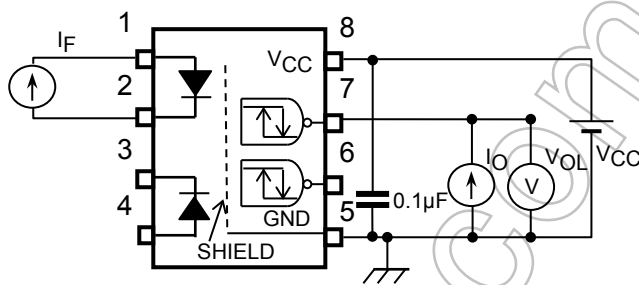
図 1: VOL 測定回路
