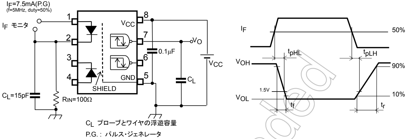
図 5: 伝達遅延時間測定回路、波形
