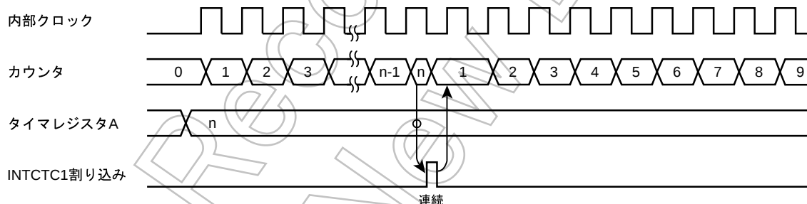
図 10-2 タイマモードタイミングチャート
