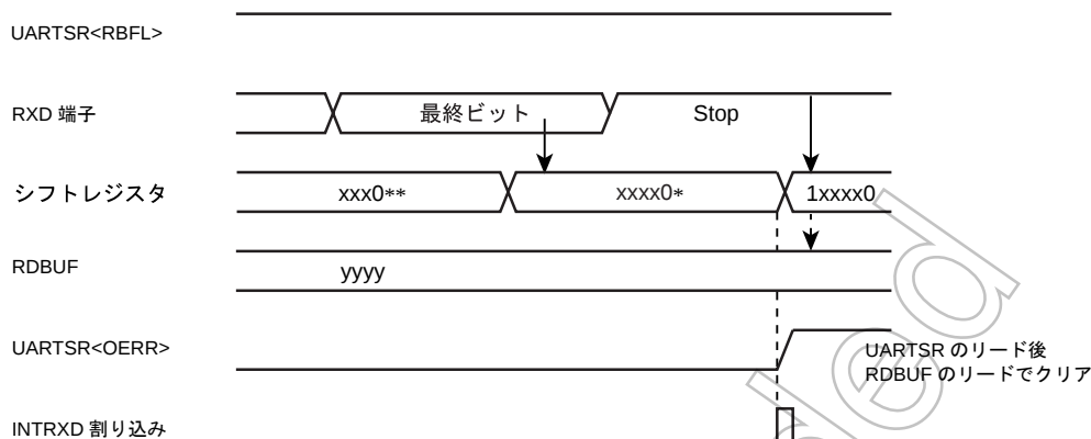
図 15-7 オーバランエラーの発生
