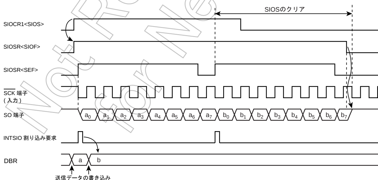
図 17-8 送信モード (例：8 ビット、1ワード転送、外部クロック)
