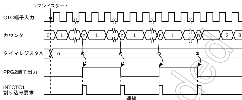
図 10-6 1 レジスタコマンドスタートモードタイミングチャート
