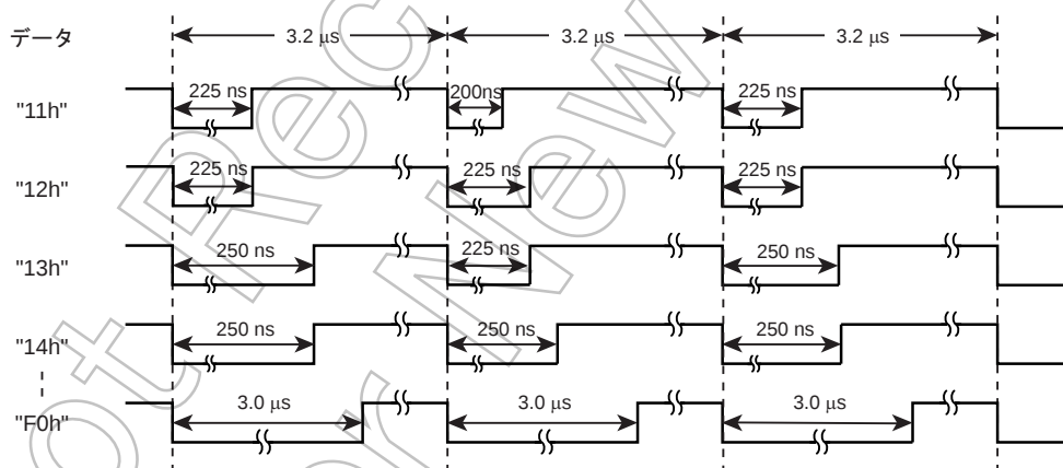
図 19-4 6 ビットモード
