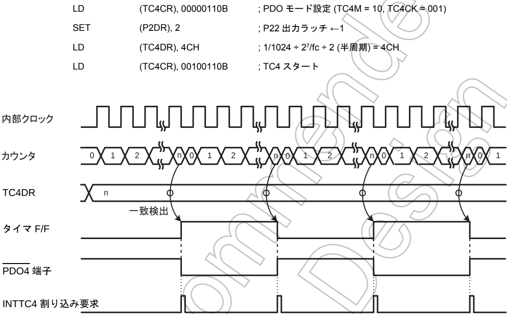
図 12-2 PDO モードタイミングチャート
