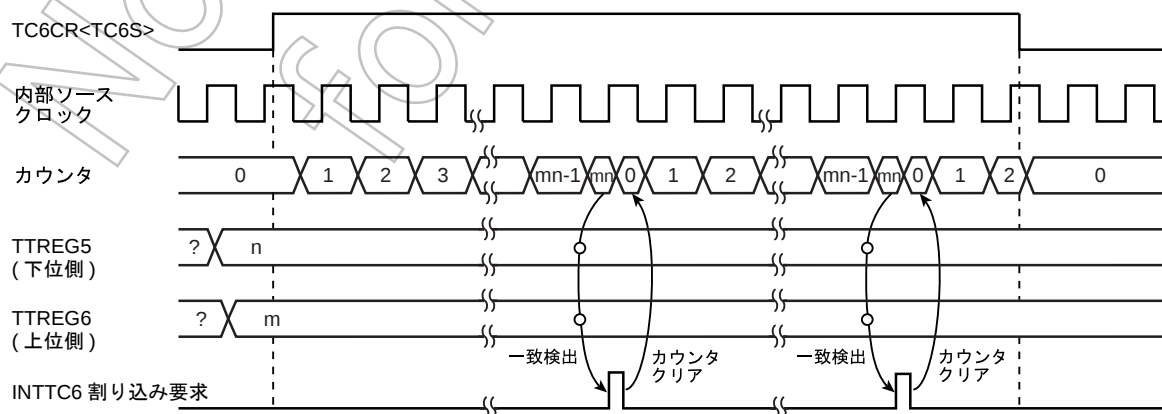
図 13-6 16 ビットタイマモードタイミングチャート (TC5 + TC6 の場合)
