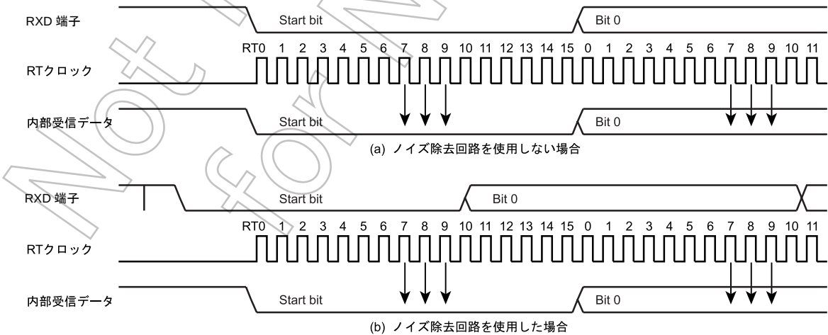
図 15-4 データのサンプリング方法
