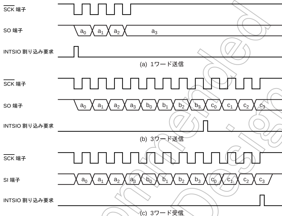
図 17-6 転送ワード数 (例 : 1 ワード = 4 ビット)
