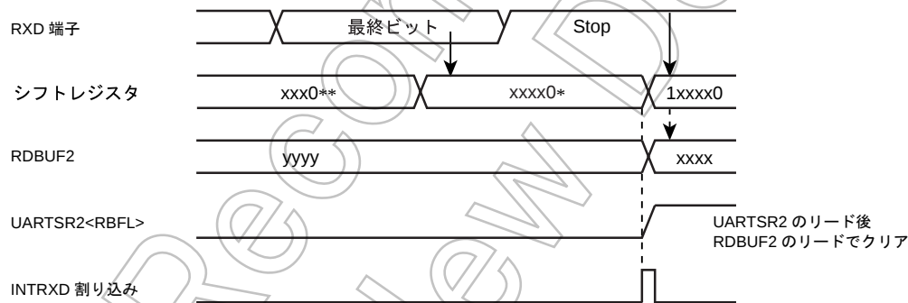
図 16-8 受信バッファフルの発生
