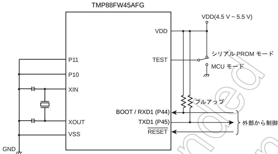
図 21-2 シリアル PROM モード端子設定
