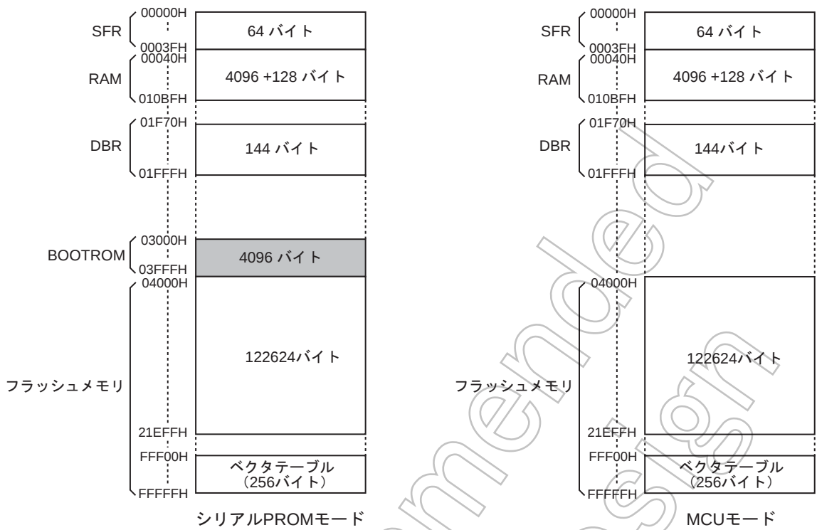
図 21-1 メモリアドレスマップ
