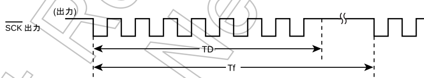
図 17-2 フレーム時間( T_f )とデータ転送時間( T_D )
