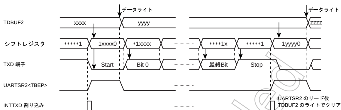
図 16-9 送信バッファエンプティの発生
