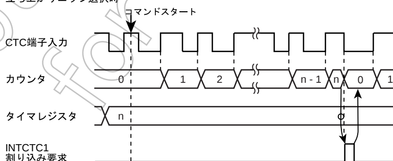
図 10-5 イベントカウンタモード タイミングチャート
