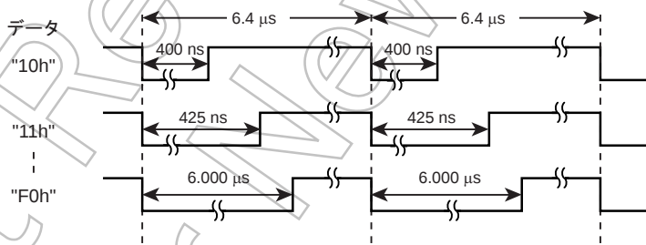
図 19-3 7 ビットモード
