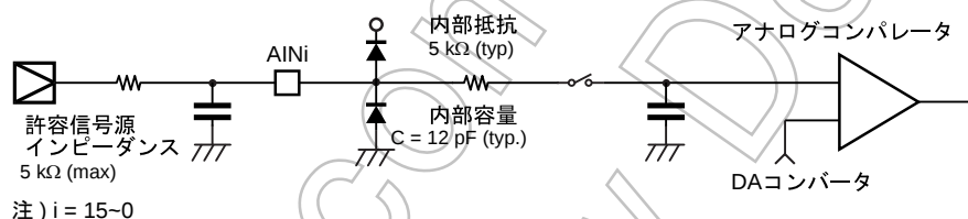
図 18-5 アナログ入力等価回路と入力端子処理例
