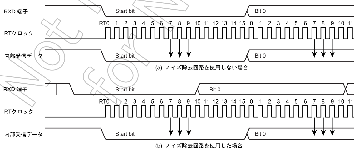
図 16-4 データのサンプリング方法
