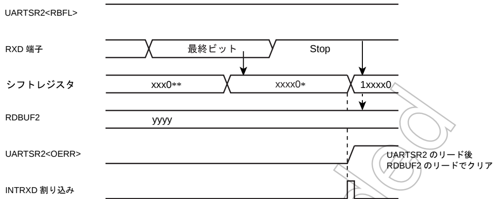
図 16-7 オーバランエラーの発生
