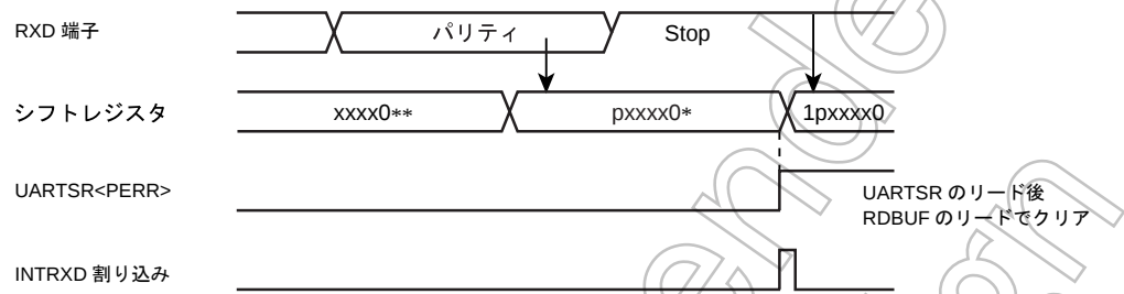
図 15-5 パリティエラーの発生
