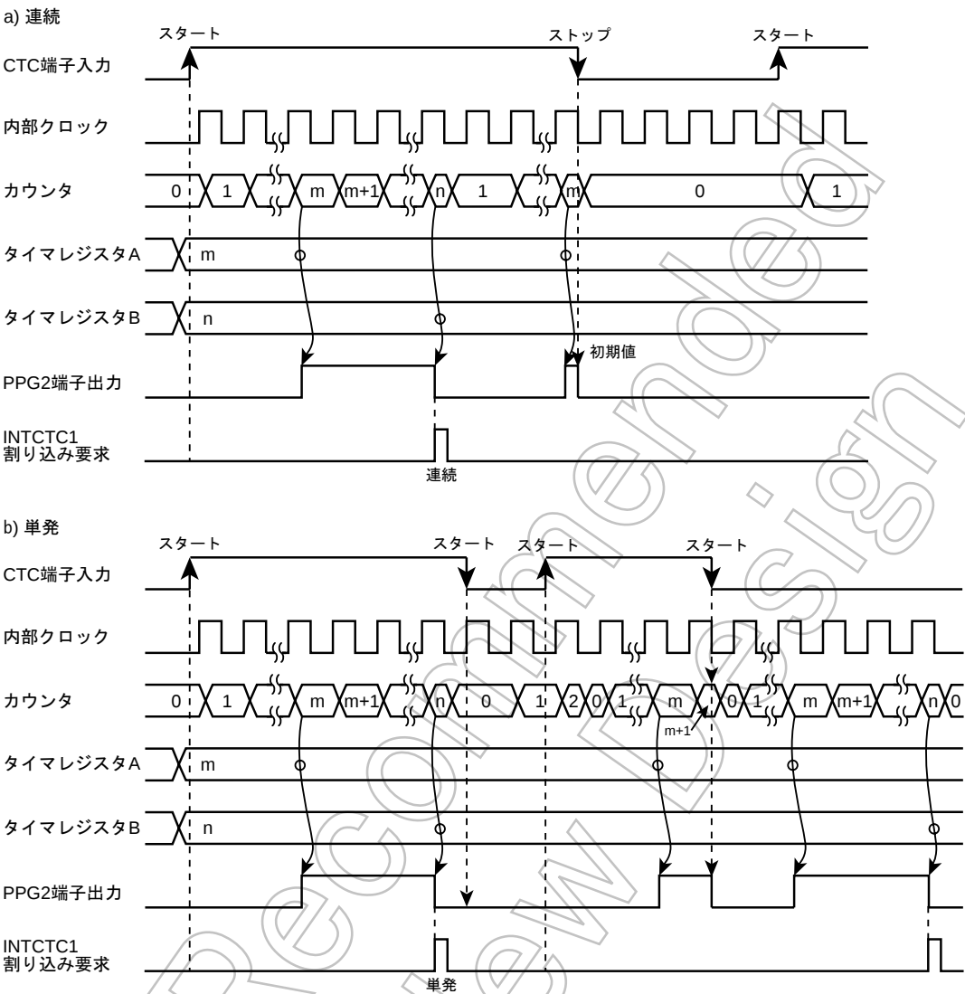
図 10-8 2 レジスタ両エッジトリガスタートモードタイミングチャート
