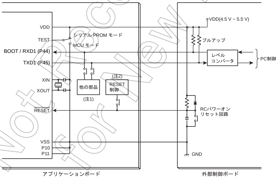
図 21-3 オンボード書き込み接続例
