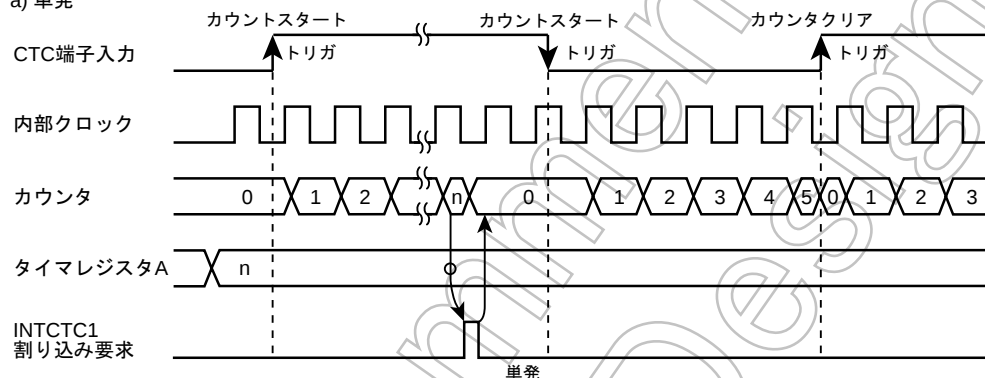
図 10-4 外部トリガモードタイミングチャート
