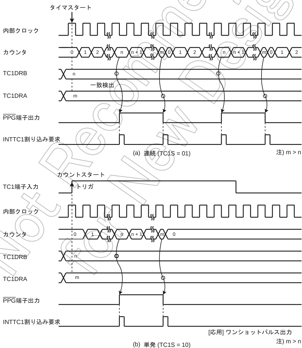
図 9-8 PPG 出力モード タイミングチャート
