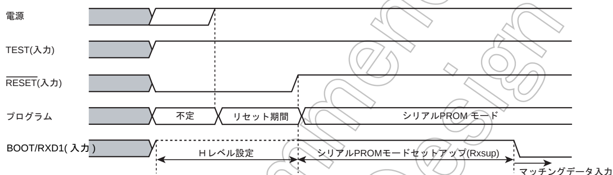
図 21-4 シリアル PROM モードタイミング
