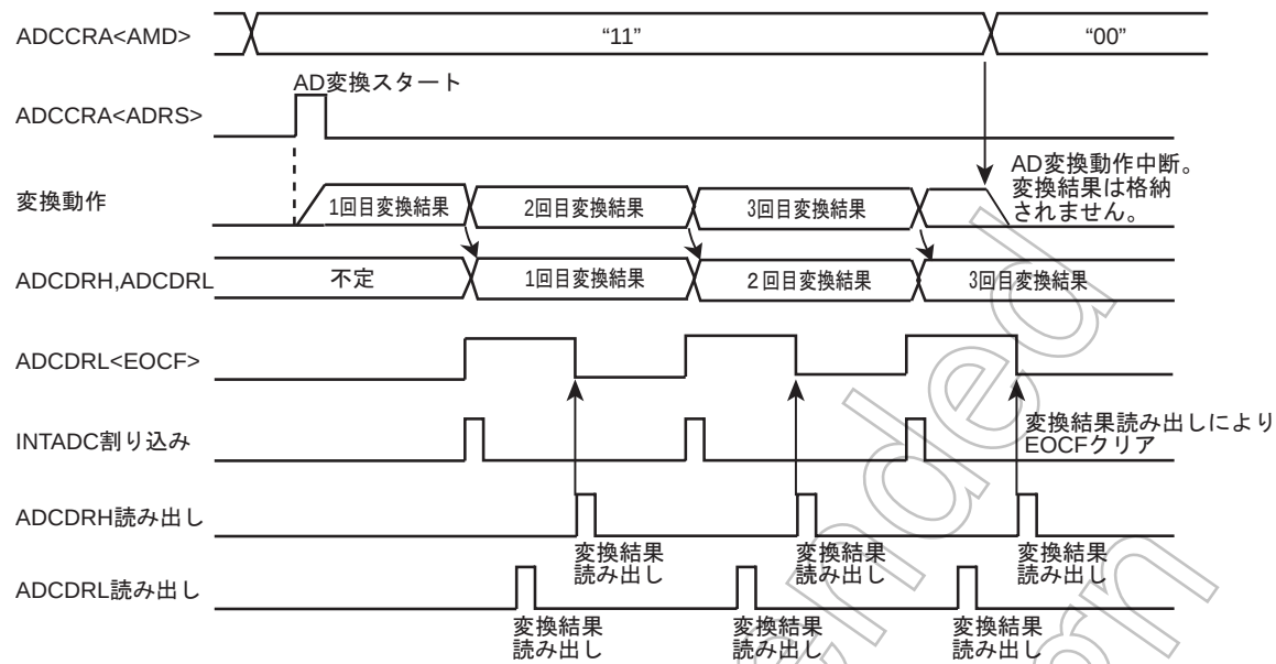
図 18-3 リピートモード
