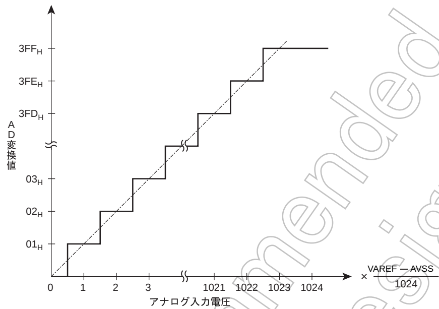
図 18-4 アナログ入力電圧と AD 変換値 (typ.) の関係
