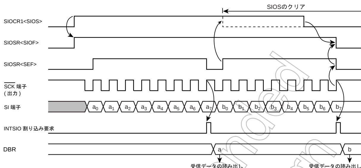
図 17-10 受信モード (例：8 ビット, 1ワード転送, 内部クロック)
