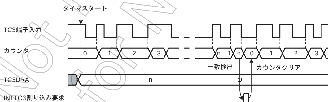
図 11-4 イベントカウンタモードタイミングチャート
