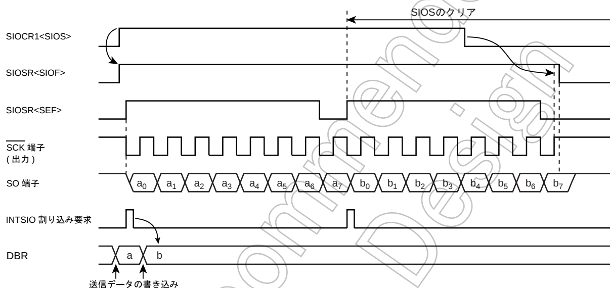
図 17-7 送信モード (例：8 ビット、1ワード転送、内部クロック)
