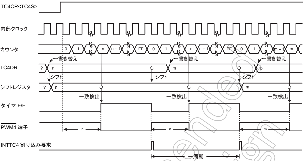
図 12-3 PWM 出力モードタイミングチャート (TC4 の例)
