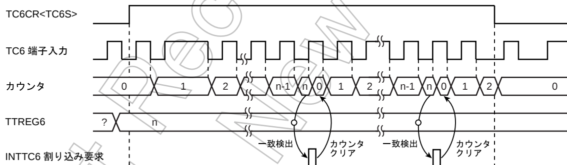
図 13-38 ビットイベントカウンタモードタイミングチャート (TC6 の場合)
