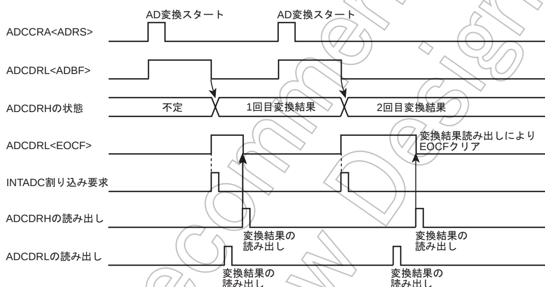
図 18-2 ソフトウェアスタートモード
