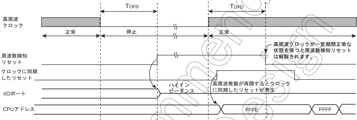
図 8-4 周波数検知リセットタイミング
