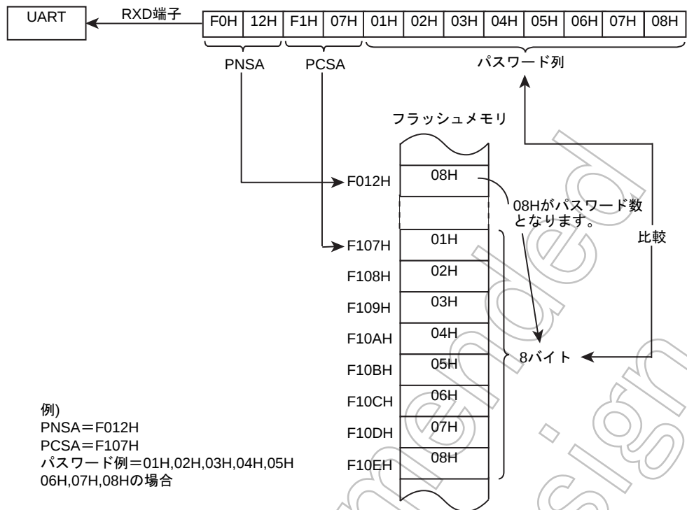
図 21-5 パスワードの比較(例)
