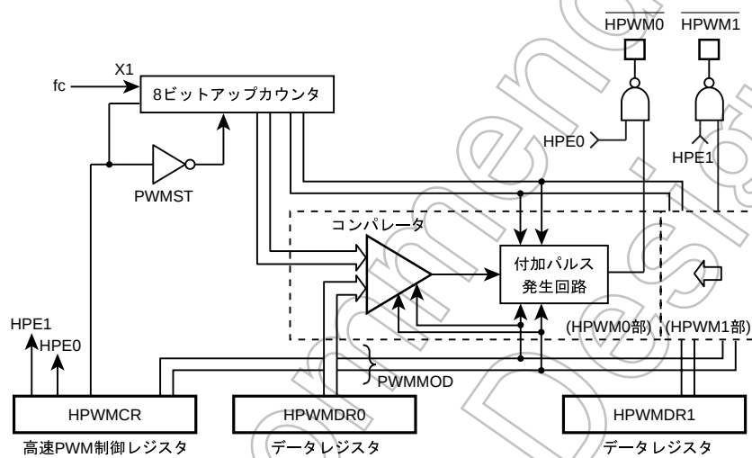
図 19-1 高速 PWM (HPWM0, HPWM1)
