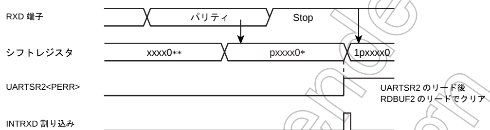
図 16-5 パリティエラーの発生
