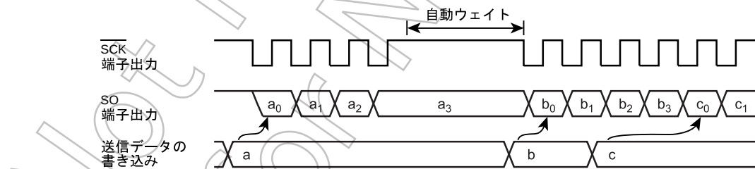
図 17-3 自動ウェイト機能 (4 ビット送信モードの場合)
