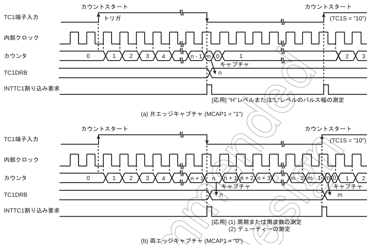
図 9-6 パルス幅測定モード
