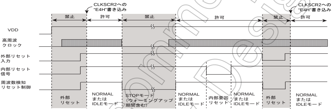
図 8-3 各モードにおける周波数検知回路動作
