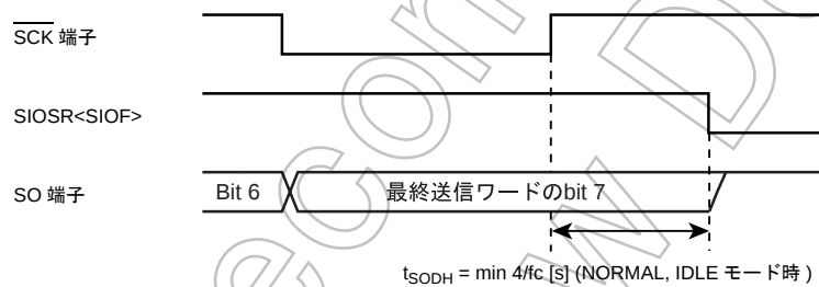
図 17-11 送受信モード (例 : 8 ビット, 1 ワード, 内部クロック)
