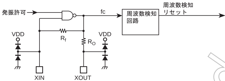
図 8-2 周波数検知回路
