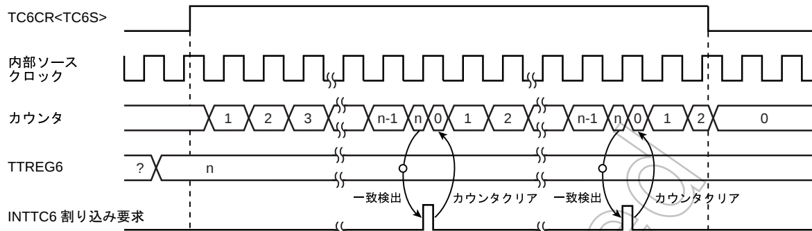
図 13-28 ビットタイマモードタイミングチャート (TC5 の場合)
