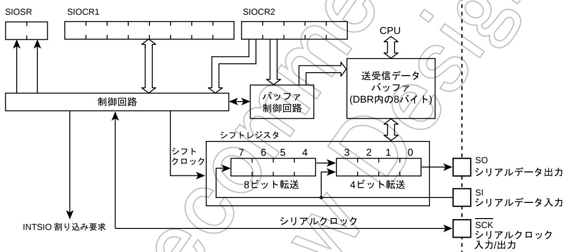
図 17-1 シリアル インタフェース
