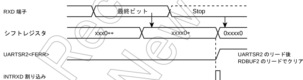
図 16-6 フレーミングエラーの発生
