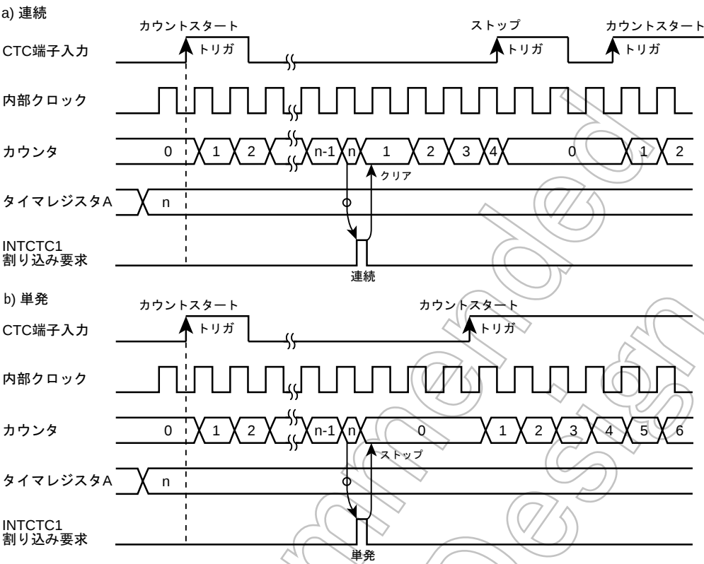
図 10-3 外部トリガモードタイミングチャート
