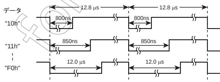
図 19-2 8 ビットモード
