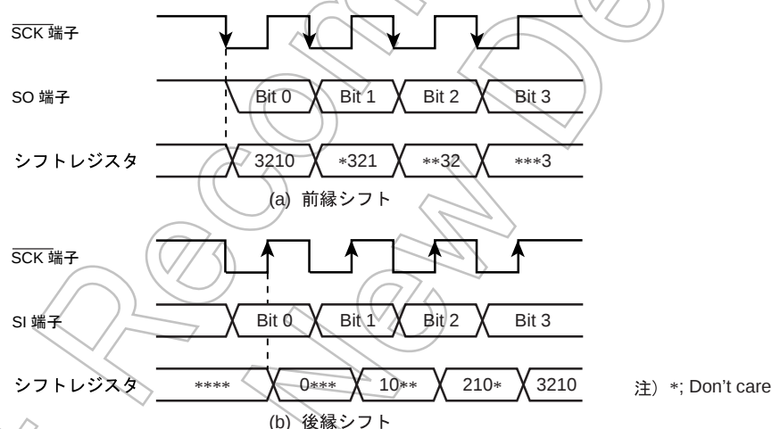
図 17-5 シフトエッジ
