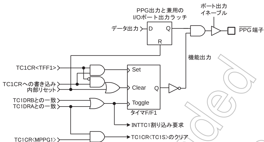
図 9-7 PPG 出力
