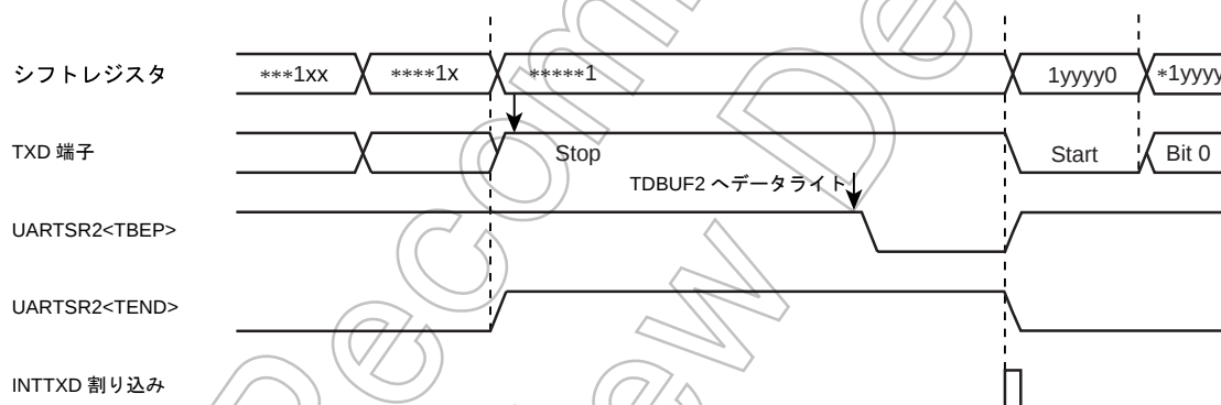
図 16-10 送信終了フラグと送信バッファエンプティの発生
