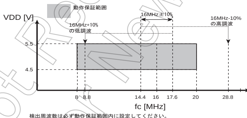
図 8-1 検出周波数範囲(初期値)
