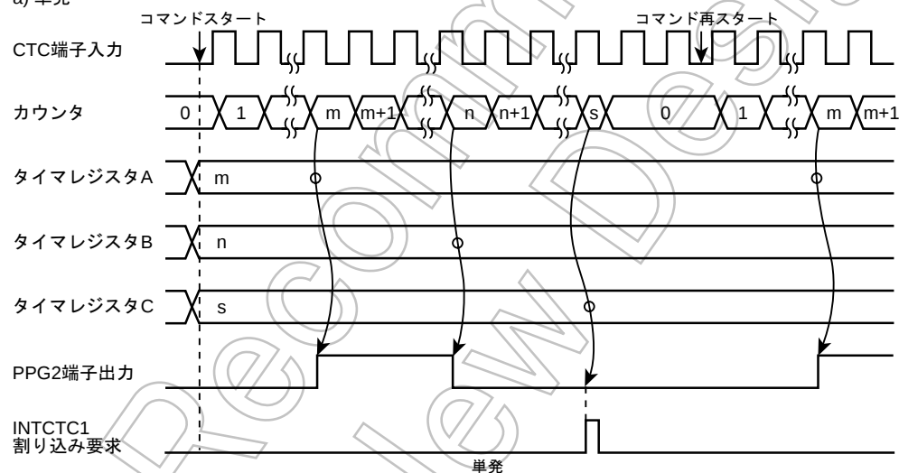
図 10-9 3 レジスタコマンドスタートモードタイミングチャート
