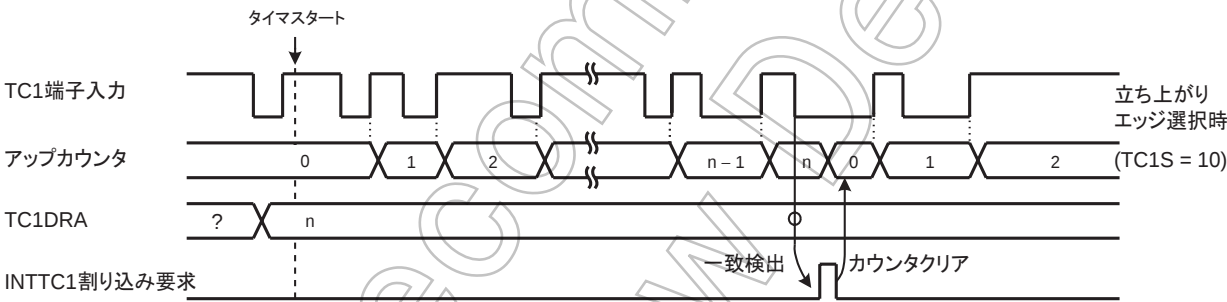
図 9-4 イベントカウンタモード タイミングチャート
