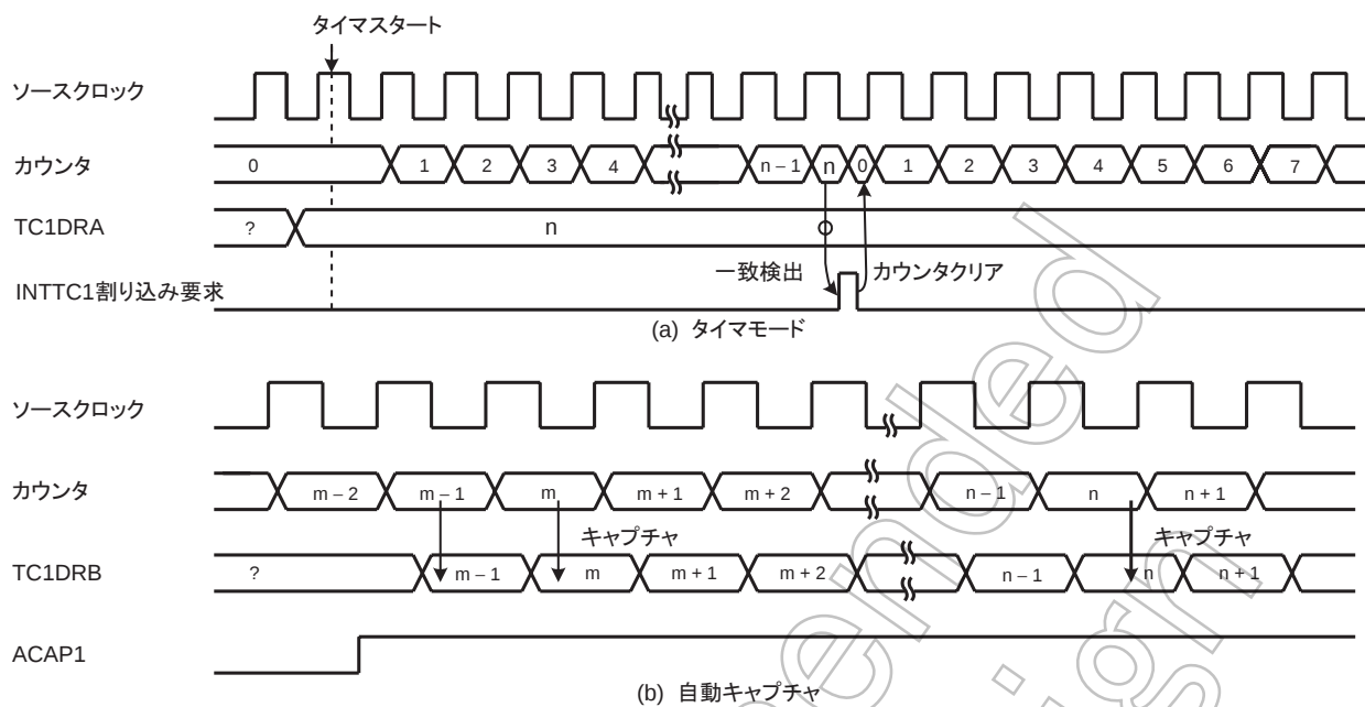
図 9-2 タイマモードタイミングチャート
