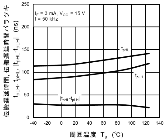
図 12.2.16 t_{pHL}, t_{pLH}, |t_{pHL} - t_{pLH}| - T_a (測定回路図12.1.7)
