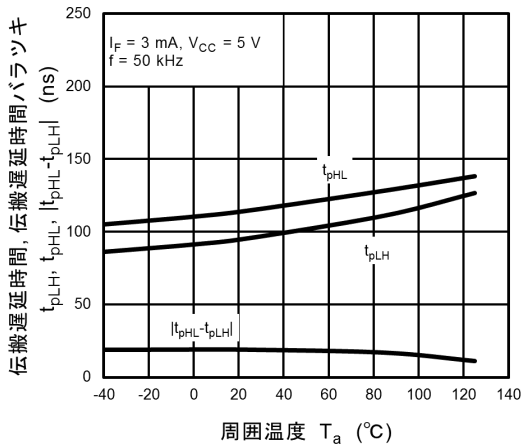
図 12.2.15 t_{pHL}, t_{pLH}, |t_{pHL} - t_{pLH}| - T_a (測定回路図12.1.7)
