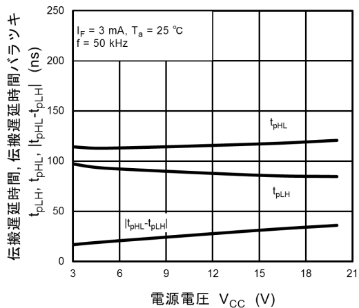
図 12.2.23 t_{pHL}, t_{pLH}, |t_{pHL} - t_{pLH}| - V_{CC} (測定回路図12.1.8)
