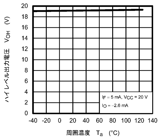
図 12.2.6 V_{OH} - T_a
