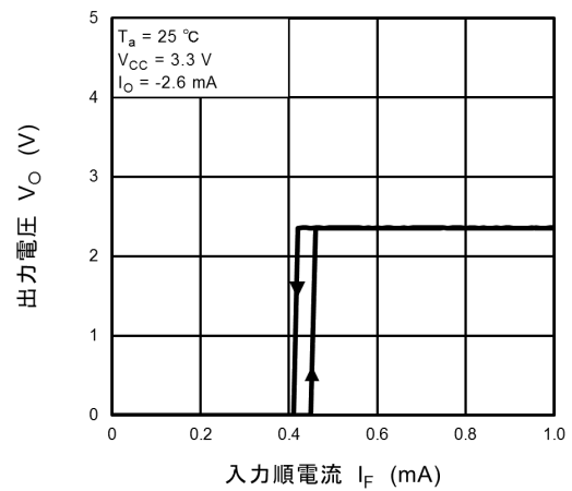
図 12.2.12 V_O - I_F
