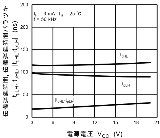
図 12.2.17 t_{pHL}, t_{pLH}, |t_{pHL} - t_{pLH}| - V_{CC} (測定回路図12.1.7)
