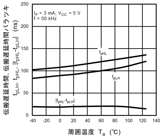
図 12.2.21 t_{pHL}, t_{pLH}, |t_{pHL} - t_{pLH}| - T_a (測定回路図12.1.8)
