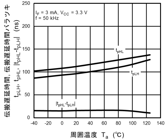
図 12.2.20 t_{pHL}, t_{pLH}, |t_{pHL} - t_{pLH}| - T_a (測定回路図12.1.8)
