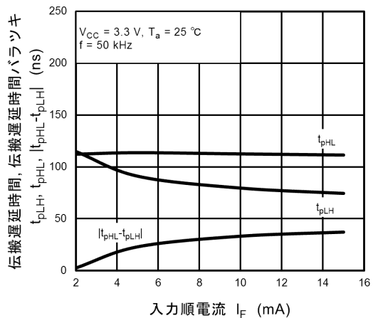
図 12.2.18 t_{pHL}, t_{pLH}, |t_{pHL} - t_{pLH}| - I_F (測定回路図12.1.7)
