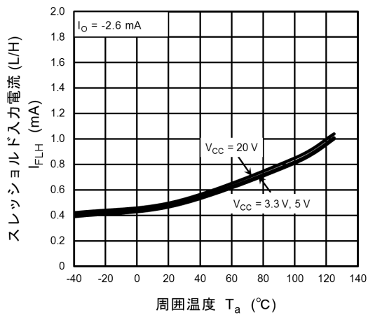
図 12.2.11 I_{FLH} - T_a
