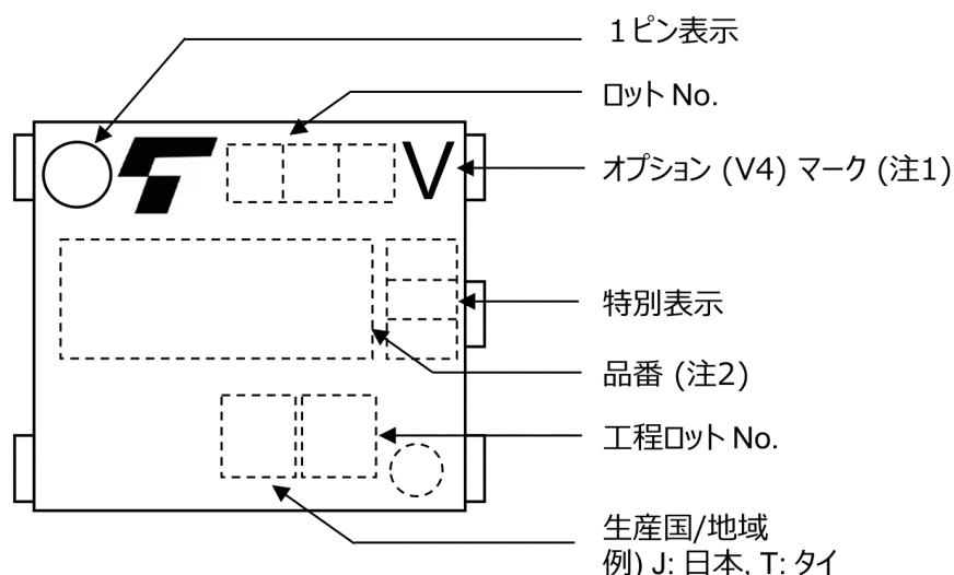
図 16.4 現品表示例
