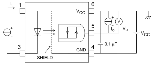
図 12.1.2 V_{OH} 測定回路
