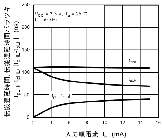
図 12.2.24 t_{pHL}, t_{pLH}, |t_{pHL} - t_{pLH}| - I_F (測定回路図12.1.8)
