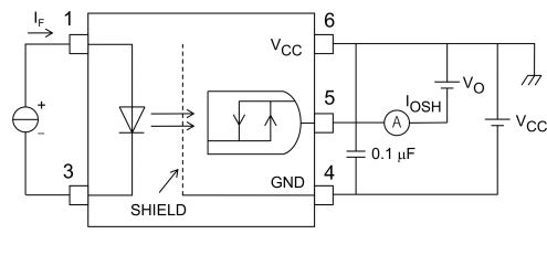
図 12.1.6 I_{OSH} 測定回路
