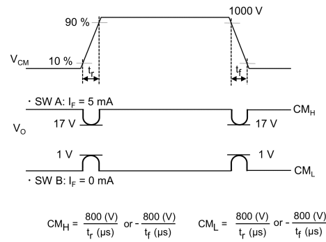
図 12.1.9 コモンモード過渡耐性測定回路, 波形
