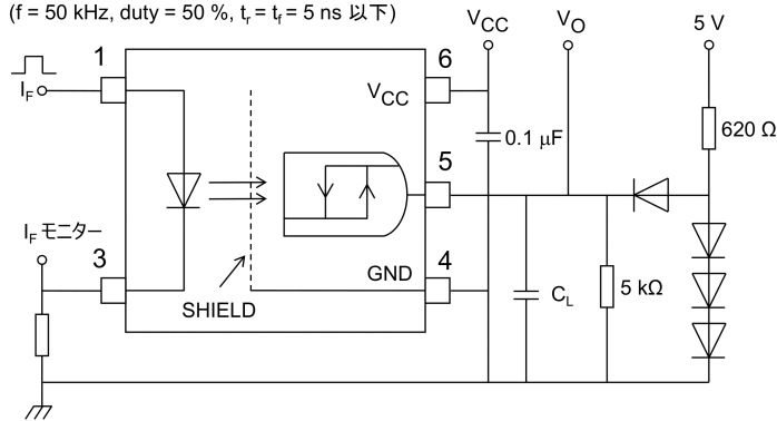
図 12.1.7 伝搬遅延時間測定回路, 波形
