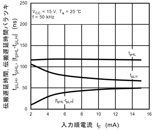
図 12.2.19 t_{pHL}, t_{pLH}, |t_{pHL} - t_{pLH}| - I_F (測定回路図12.1.7)
