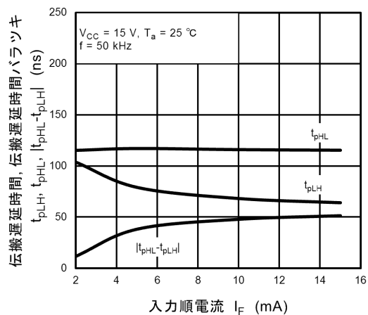
図 12.2.25 t_{pHL}, t_{pLH}, |t_{pHL} - t_{pLH}| - I_F (測定回路図12.1.8)
