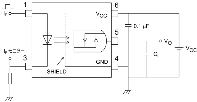
図 12.1.8 伝搬遅延時間測定回路, 波形
