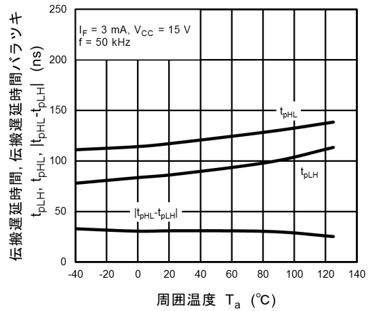
図 12.2.22 t_{pHL}, t_{pLH}, |t_{pHL} - t_{pLH}| - T_a (測定回路図12.1.8)
