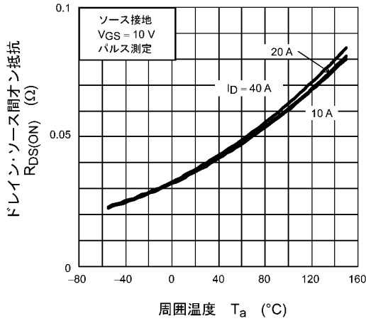
図 8.7 R_{DS(ON)} - T_a
