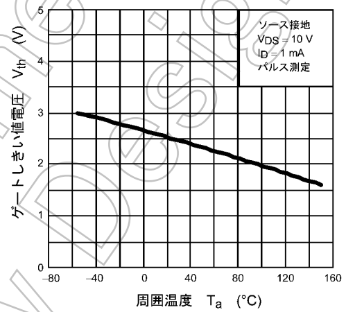
図 8.10 V_{th} - T_a
