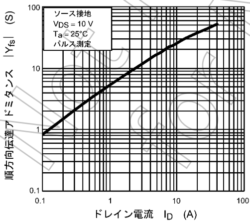
図 8.5 |Y_{fs}| - I_D
