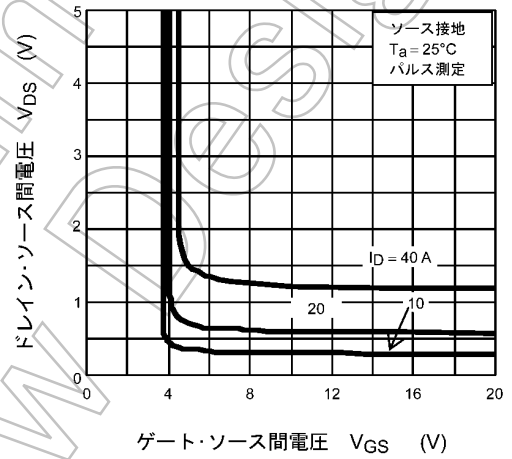
図 8.4 V_{DS} - V_{GS}
