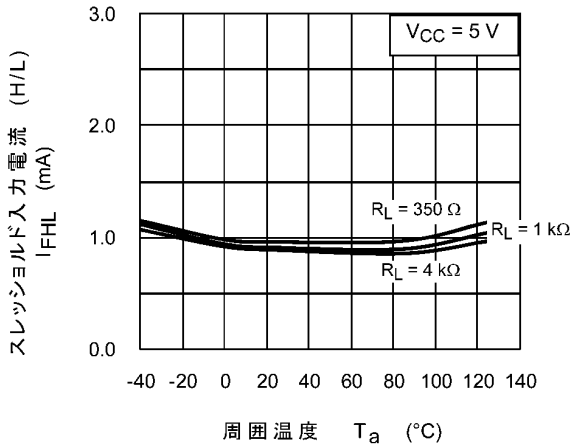
図 12.2.7 I_{FHL} - T_a
