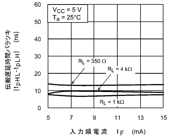
図 12.2.16 |t_{pHL} - t_{pLH}| - I_F
