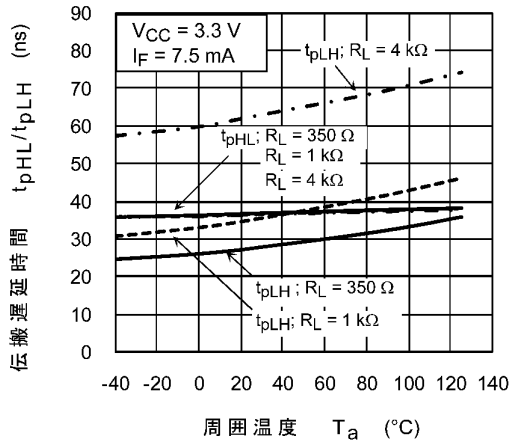
図 12.2.13 t_{pHL}, t_{pLH} - T_a
