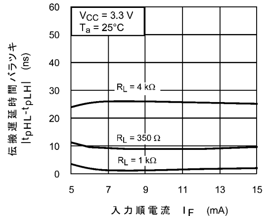
図 12.2.18 |t_{pHL} - t_{pLH}| - I_F
