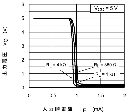
図 12.2.5 V_O - I_F
