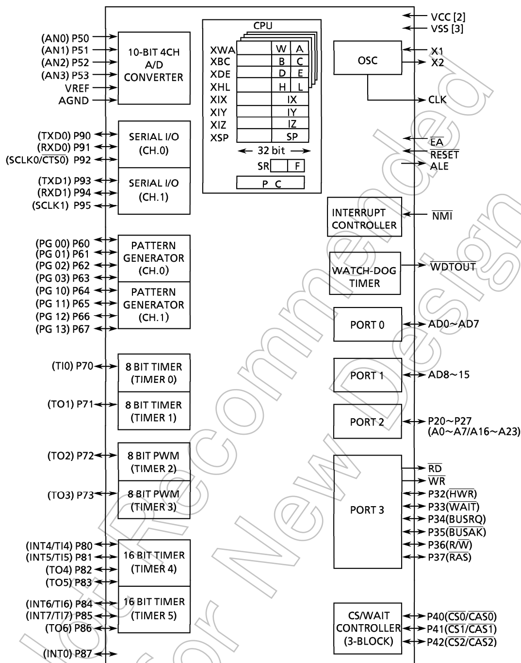
図1 TMP96C041Bブロック図
