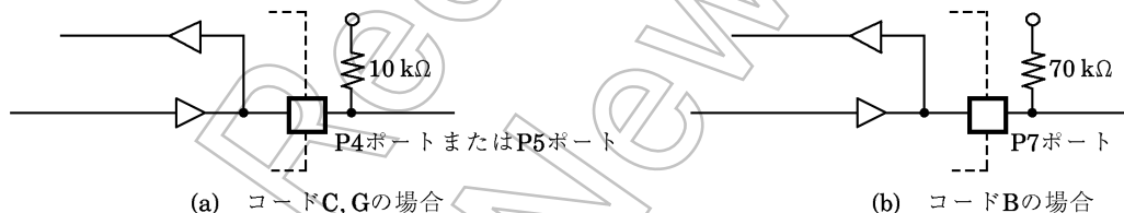
図1-3. 入出力回路のコードと外付け回路
