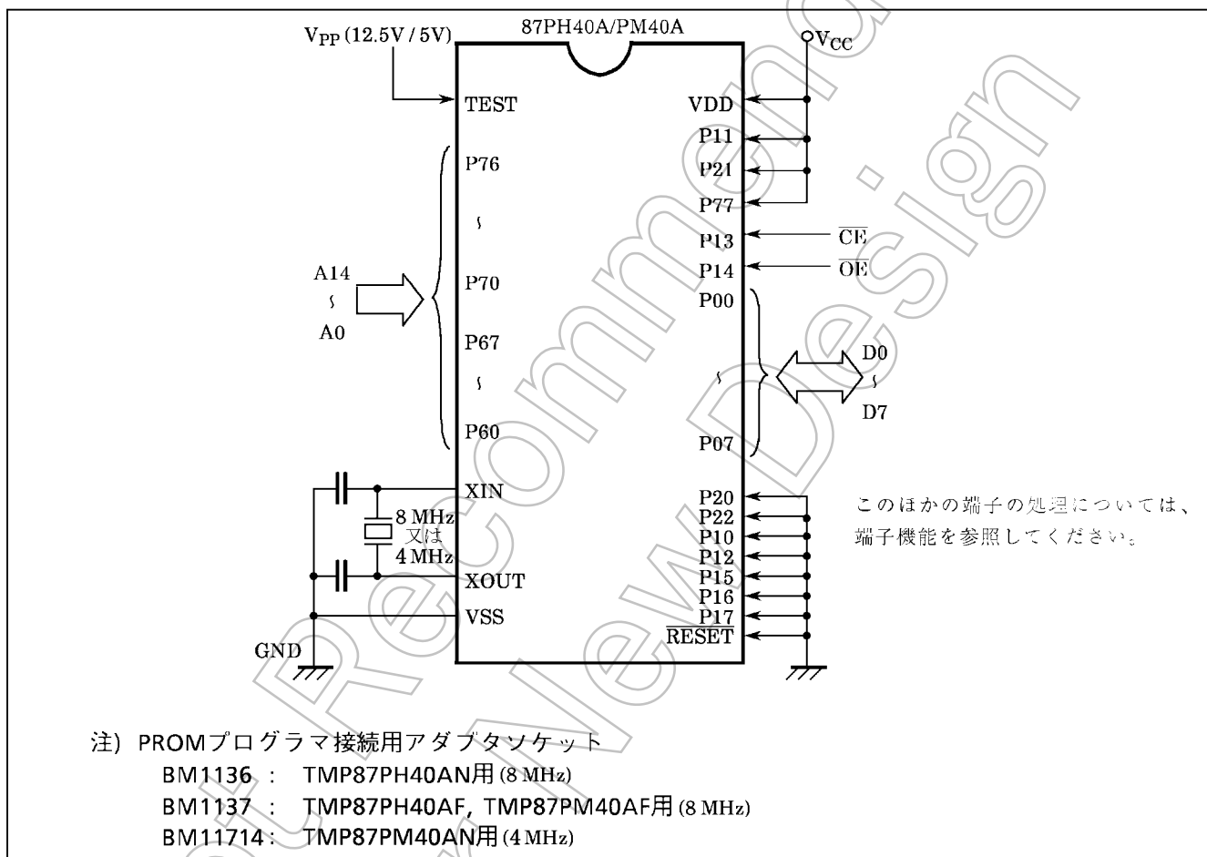
図1-4. PROMモードの設定
