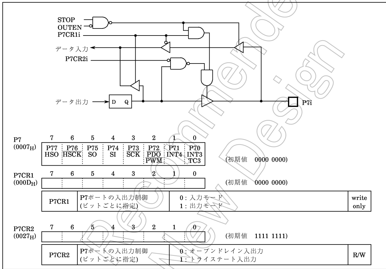
図2-8. P7ポートとP7ポート入出力制御レジスタ
