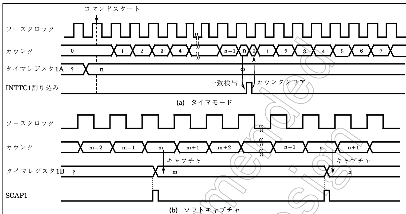
図2-15. タイマモードタイミングチャート
