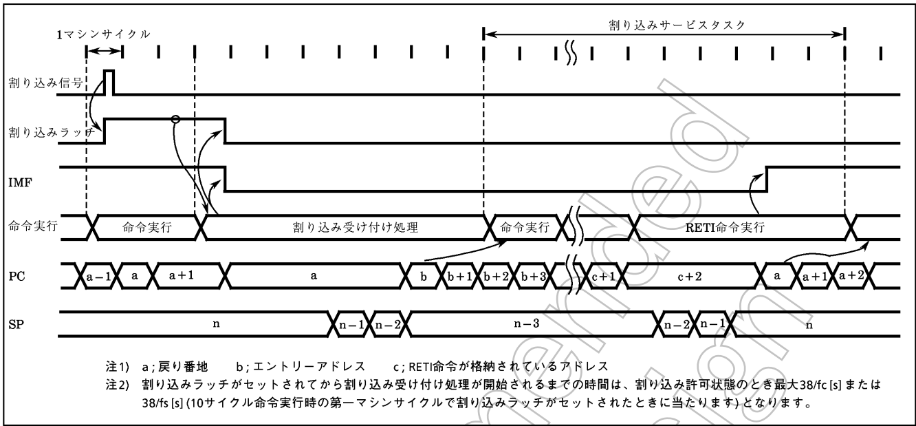
図1-24. 割り込み受け付け処理/割り込みリターン命令タイミングチャート
