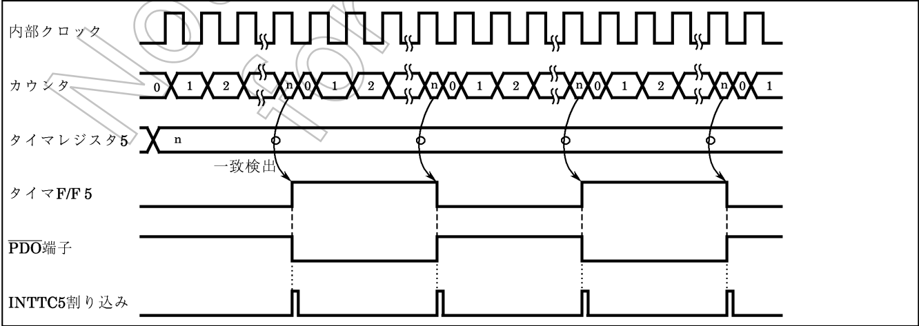
図2-30. PDOモード タイミングチャート
