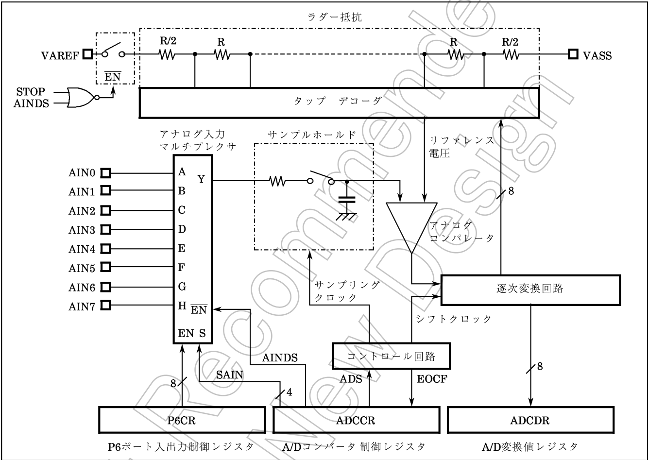
図2-46. A/Dコンバータ (ADC)
