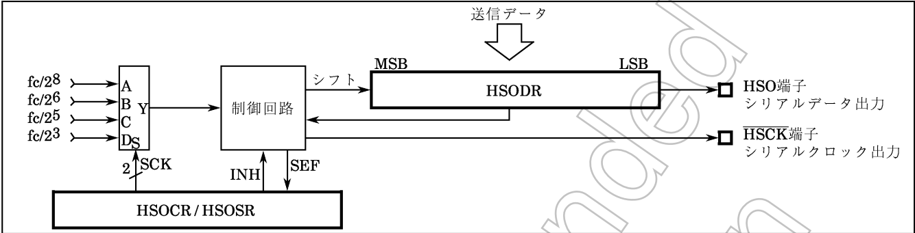
図2-43. 高速シリアル出力
