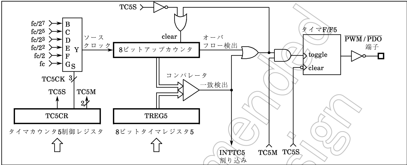
図2-28. タイマカウンタ5 (TC5)
