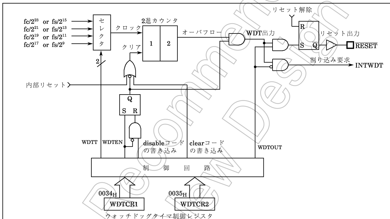
図1-27. ウォッチドッグタイマの構成
