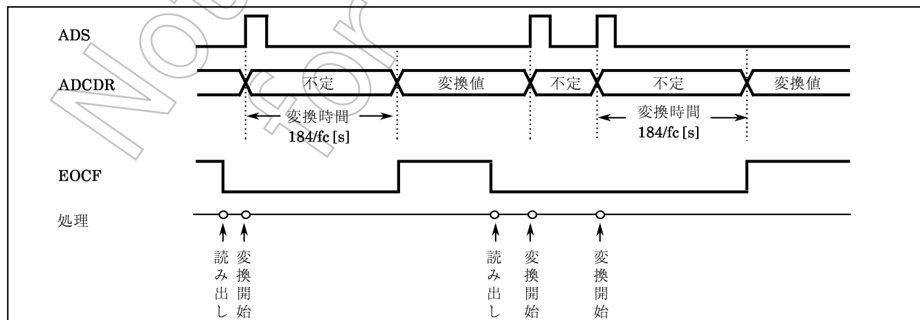
図2-49. A/D変換動作
