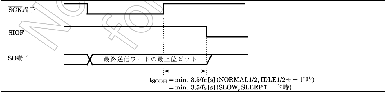
図2-39. 送信終了時の送信データ保持時間
