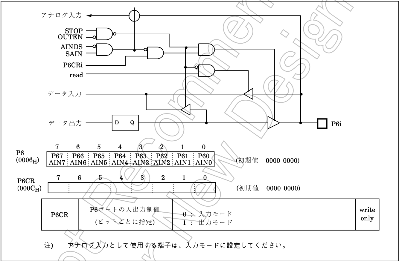
図2-7. P6ポートとP6ポート入出力制御レジスタ
