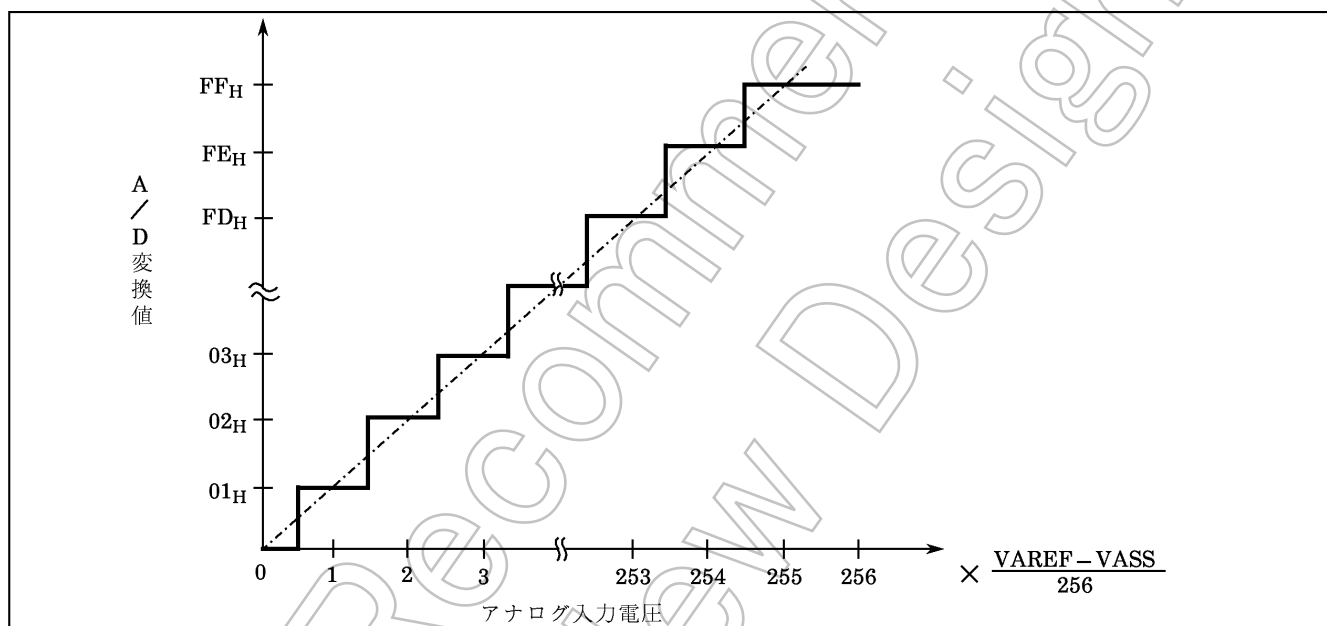
図2-50. アナログ入力電圧とA/D変換値 (typ.) の関係
