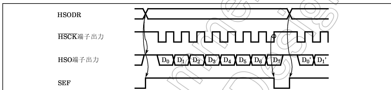
図2-45. 高速シリアル出力タイミング
