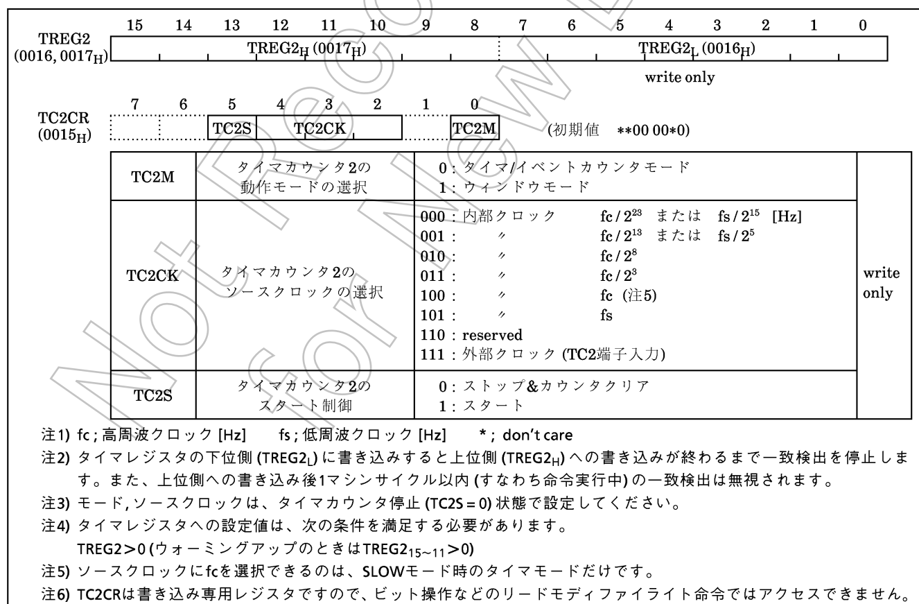
図2-23. タイマカウンタ2のタイマレジスタと制御レジスタ
