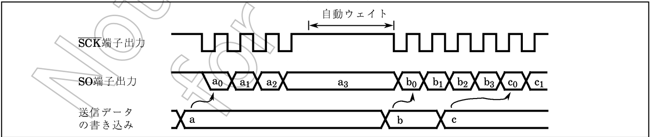
図2-35. クロックソース (内部クロック)
