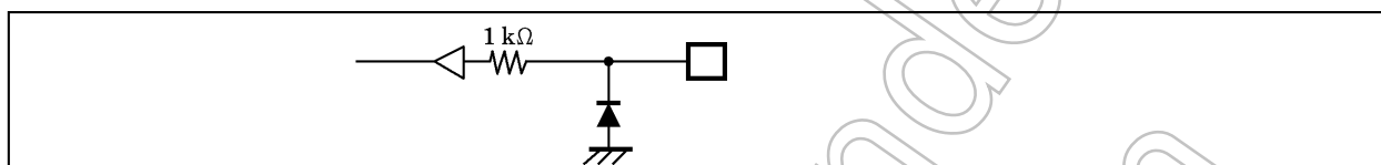
図1-2. TEST 端子
