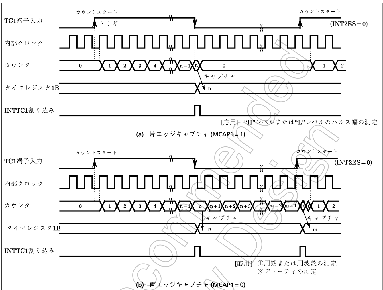
図2-19. パルス幅測定モード
