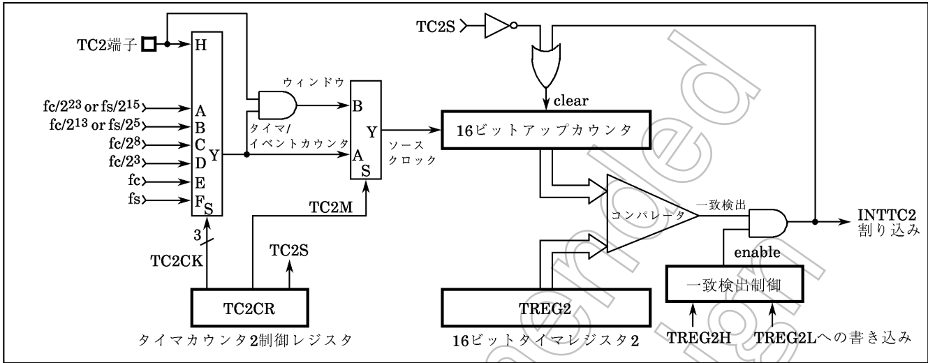
図2-22. タイマカウンタ2 (TC2)
