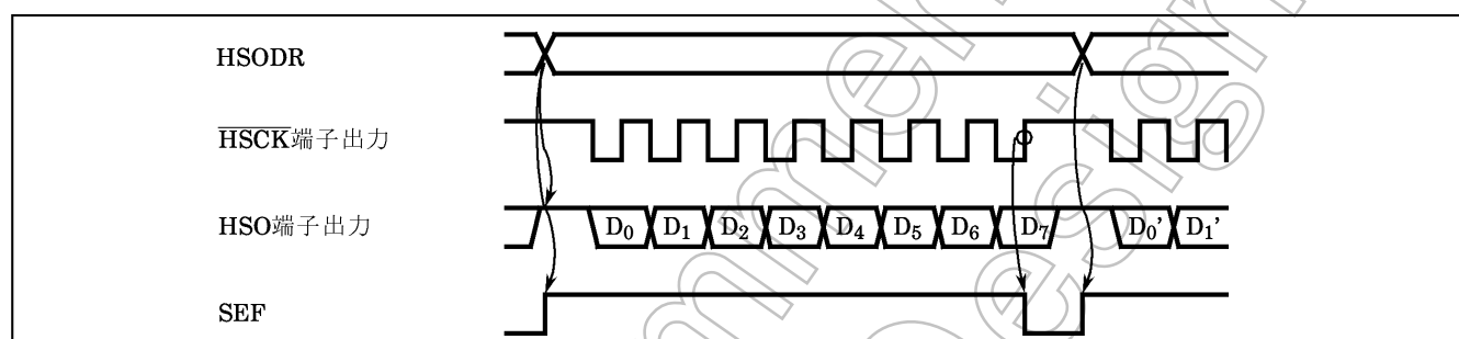
図2-47. 高速シリアル出力タイミング
