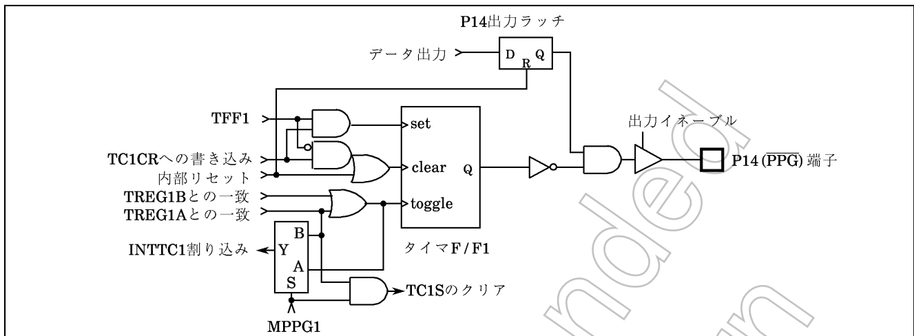
図2-20. PPG出力
