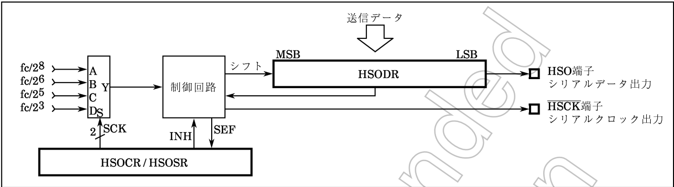
図2-45. 高速シリアル出力
