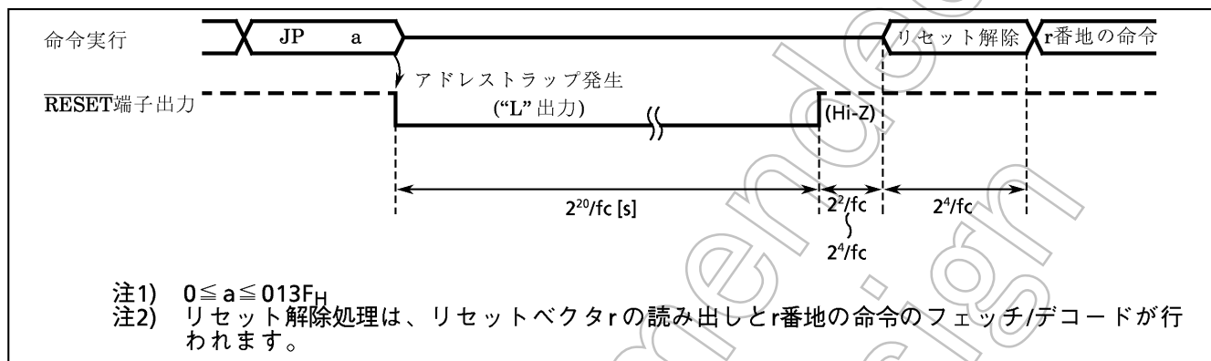
図1-31. アドレストラップリセット
