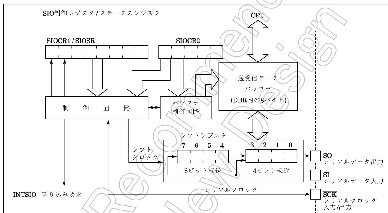
図2-32. シリアルインタフェース
