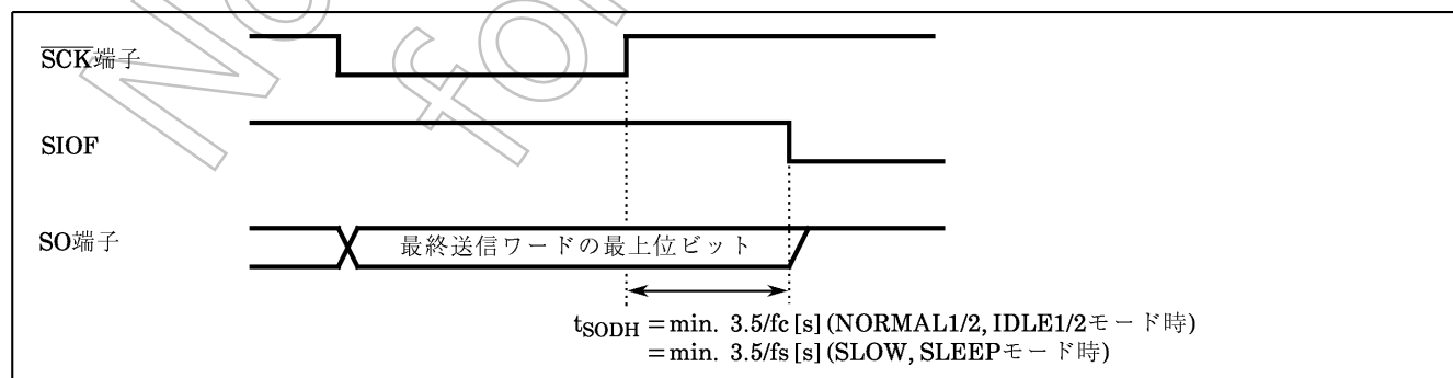
図2-39. 送信終了時の送信データ保持時間
