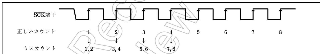
図2-44. リンギングノイズによるカウント (例) (8ビット受信モードの場合)
