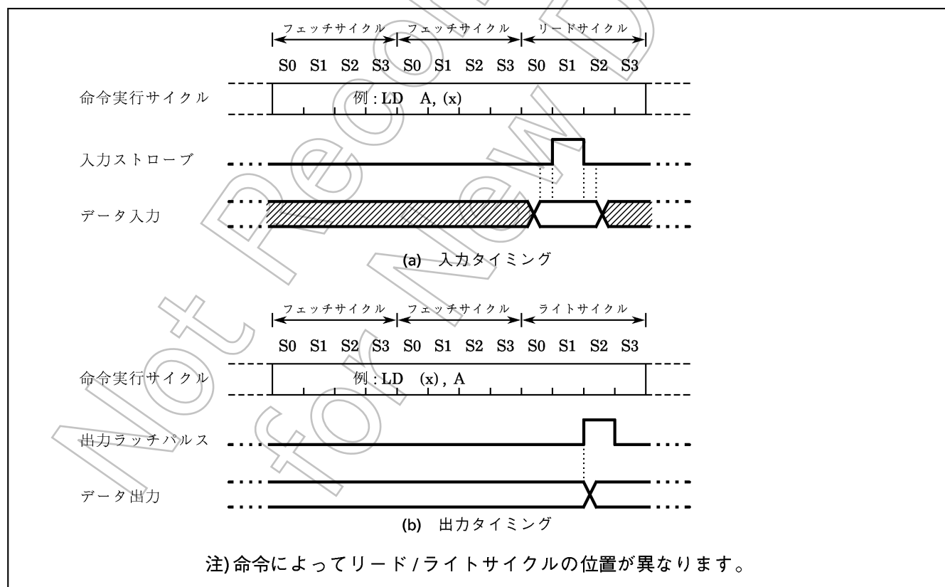
図2-2. 入出力タイミング (例)
