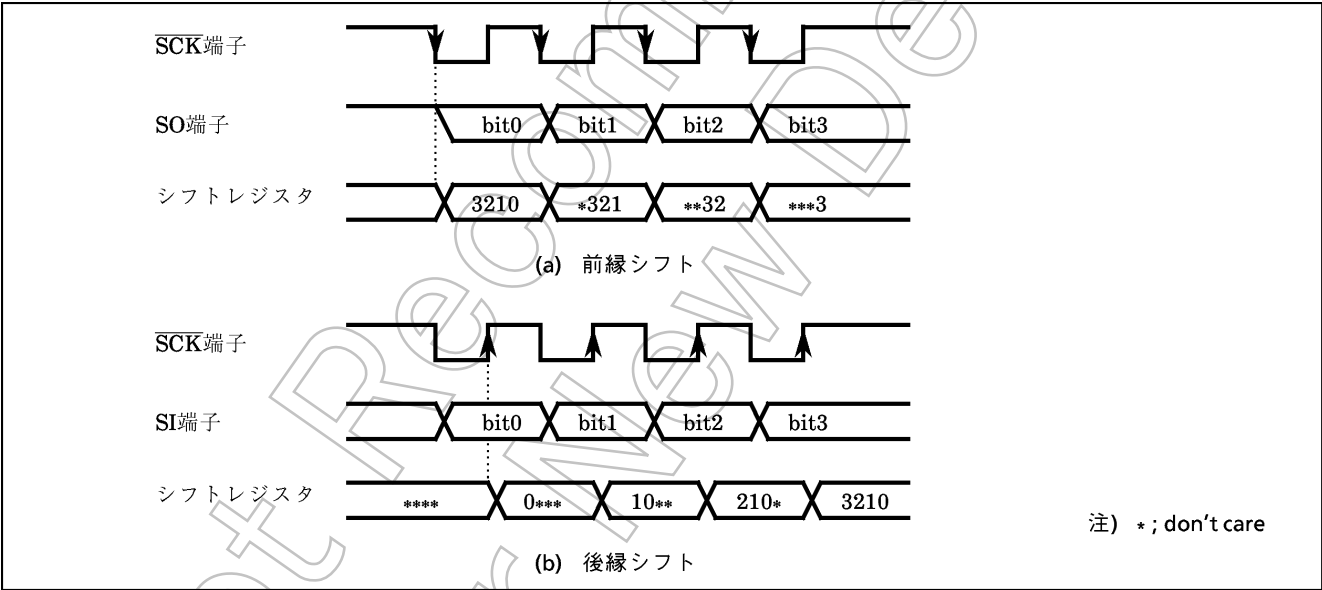
図2-36. シフトエッジ
