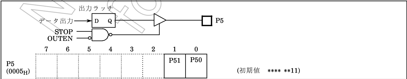
図2-6. P5ポート
