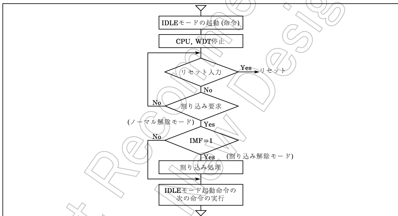
図1-19. IDLEモード
