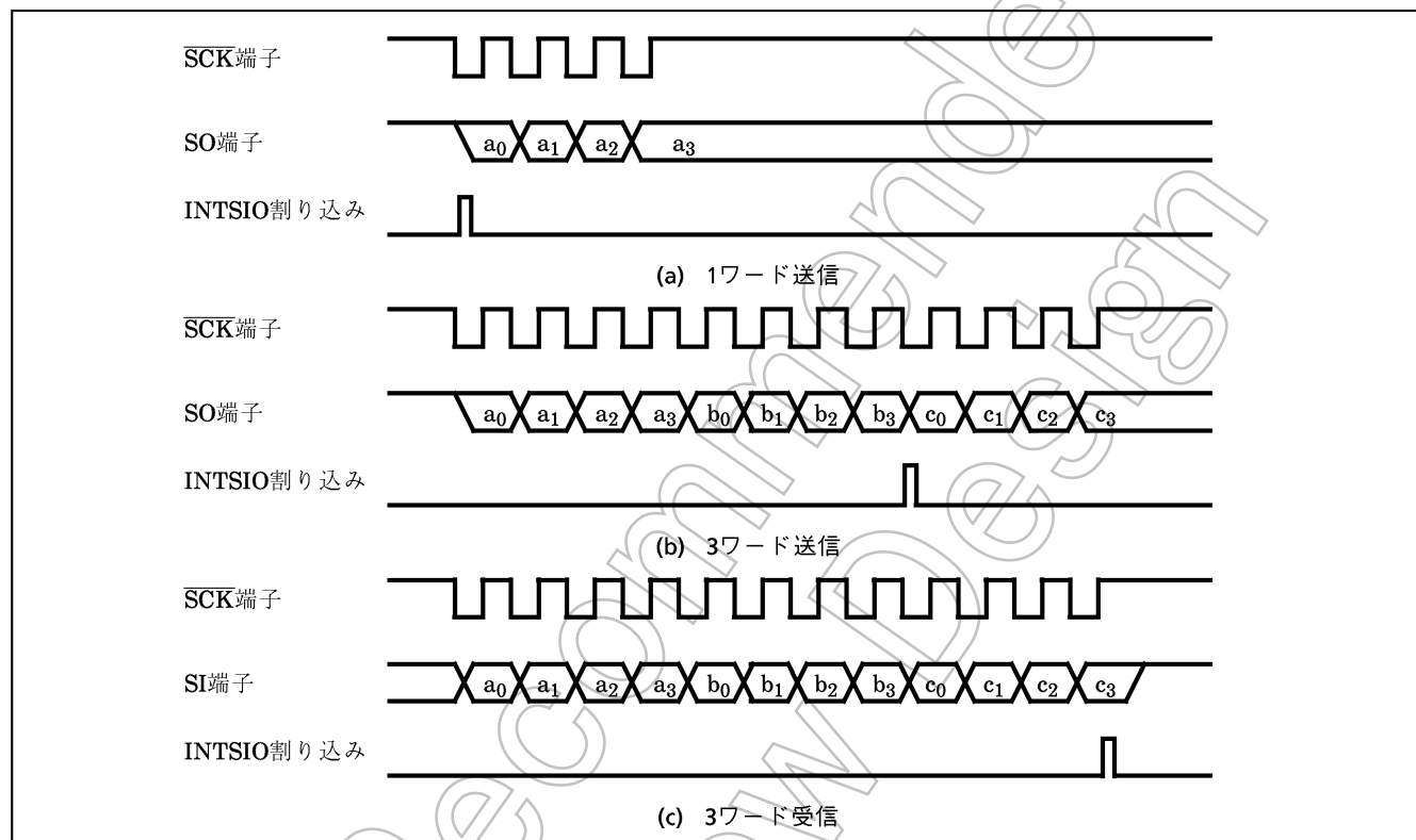
図2-37. 転送ワード数 (例: 1ワード = 4ビット)
