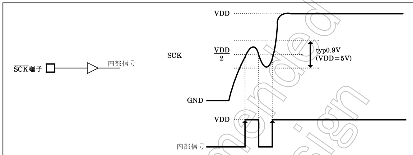
図2-43. リンギングノイズ (例)
