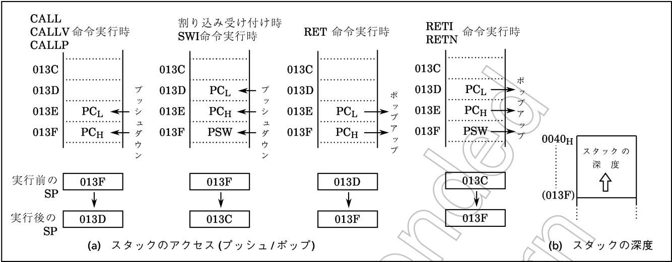
図1-8. スタック
