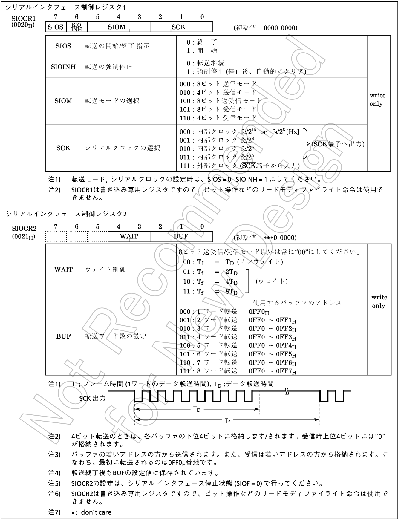
図2-33. シリアルインタフェース制御レジスタ
