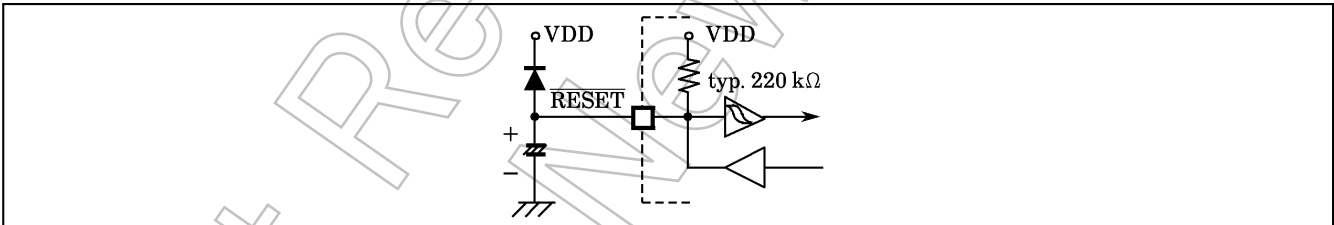
図1-30. 簡易型パワーオンリセット回路
