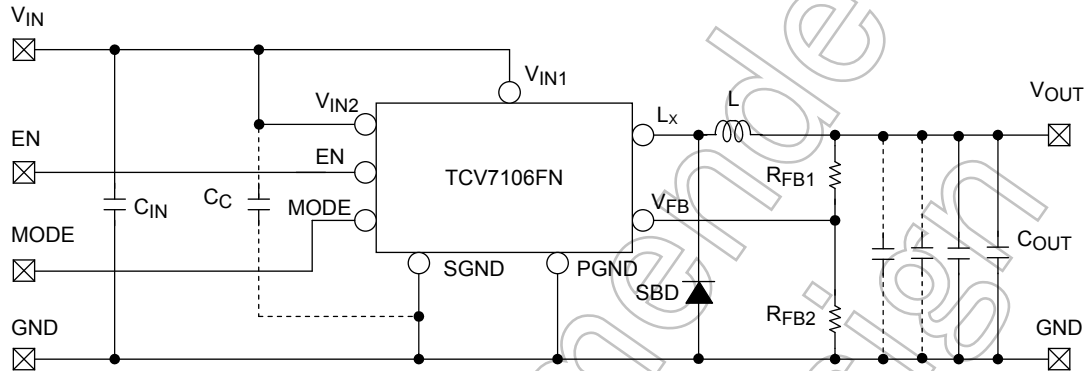
図 1 TCV7106FN 応用回路例
