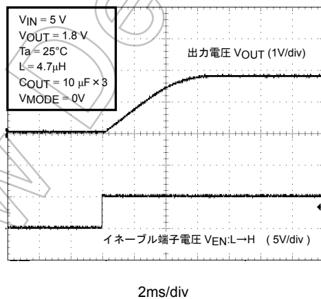
起動特性 (チョップパモード ソフトスタート時間)
