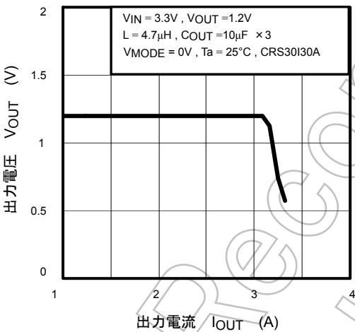
過電流特性 (チョップモード)
