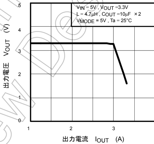
過電流特性 (同期整流モード)
