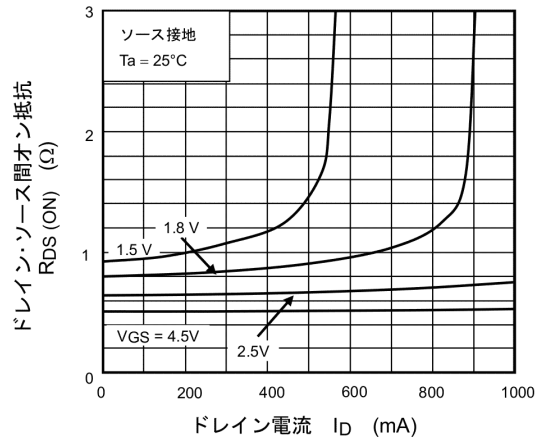
図 7.4 R_{DS(ON)} - I_D
