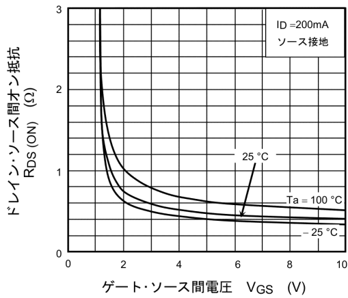
図 7.3 R_{DS(ON)} - V_{GS}
