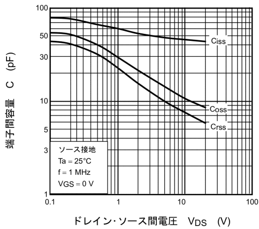
図 7.9 C - V_{DS}
