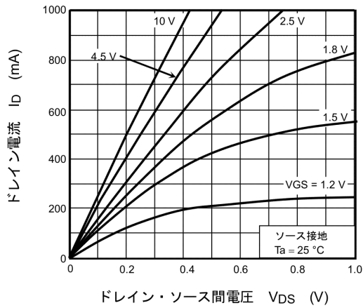
図 7.1 I_D - V_{DS}
