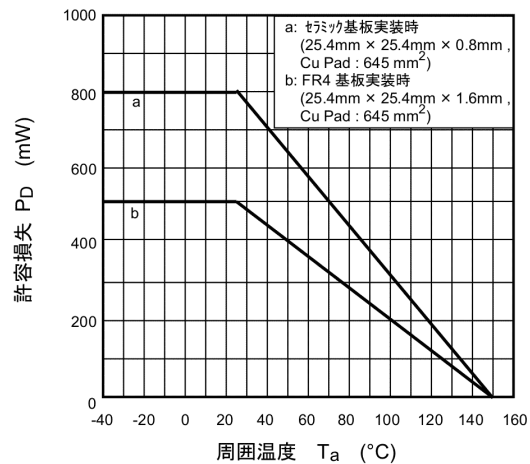
図 7.12 P_D - T_a
