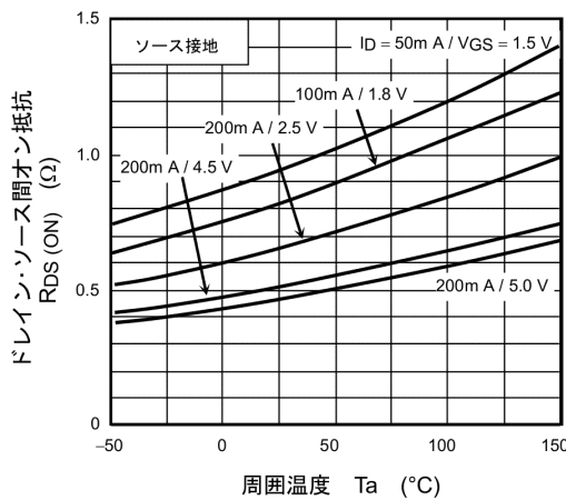
図 7.5 R_{DS(ON)} - T_a
