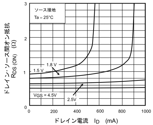
図 7.4 R_{DS(ON)} - I_D
