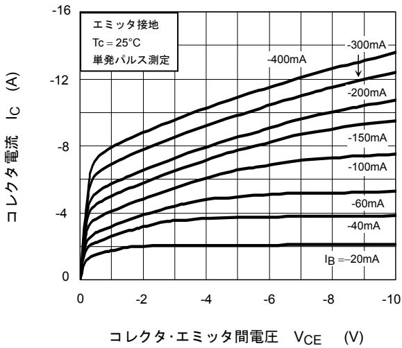
I_C - V_{CE}
