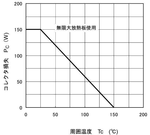
P_C - T_c
