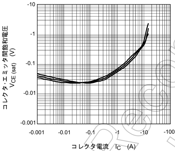
V_{CE(sat)} - I_C
