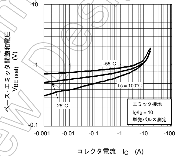
V_{BE(sat)} - I_C
