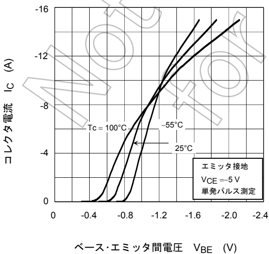
I_C - V_{BE}
