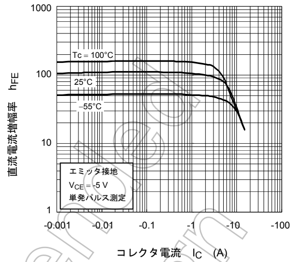
h_{FE} - I_C
