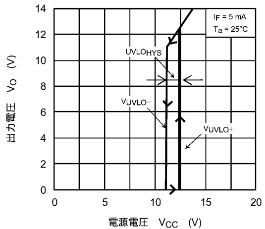
図 13.2.12 VO(VUVLO) - VCC
