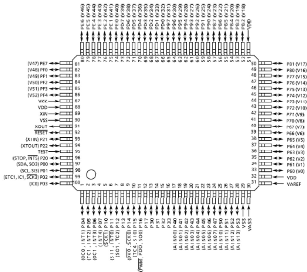
パッケージ名称 QFP100-P-1420-0.65A
