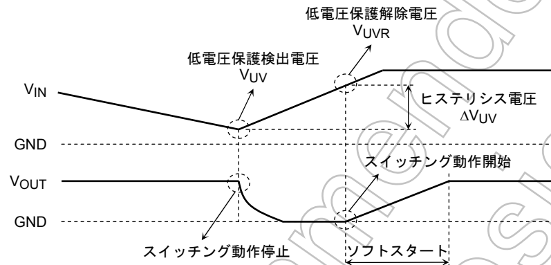
図 4 低電圧保護動作
