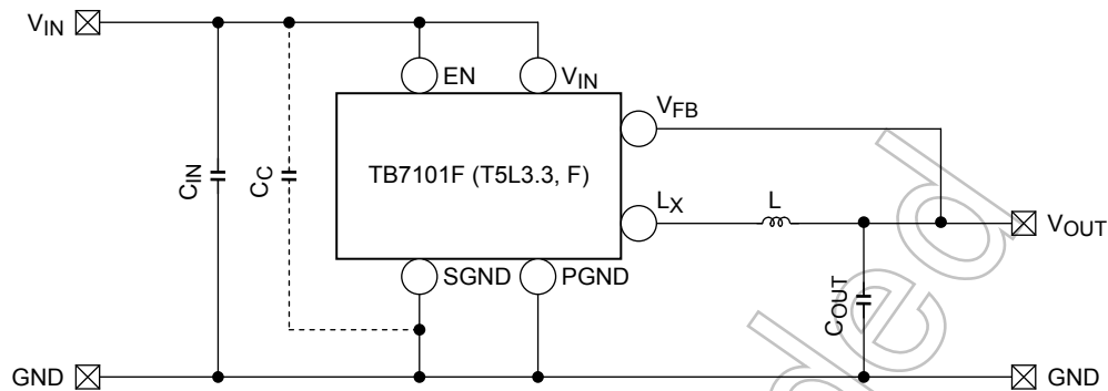
図 1 TB7101F (T5L3.3, F) 応用回路例
