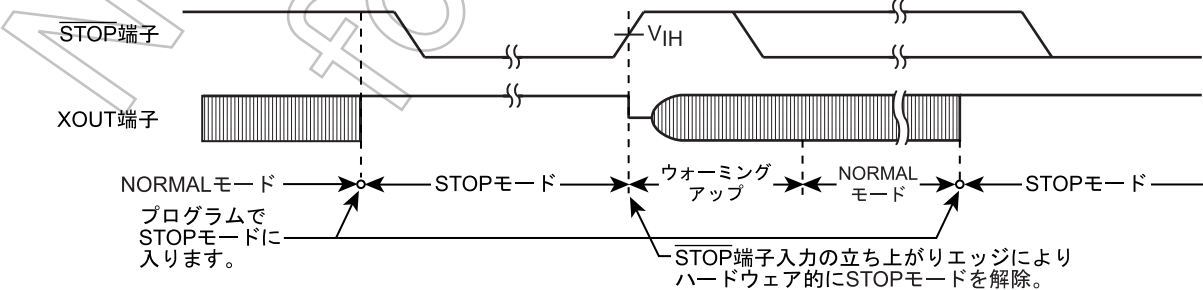
図 2-8 エッジ解除モード
