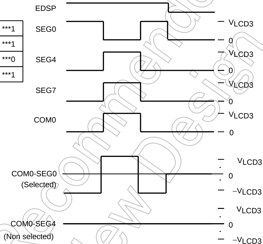
図 15-11 スタティック駆動
