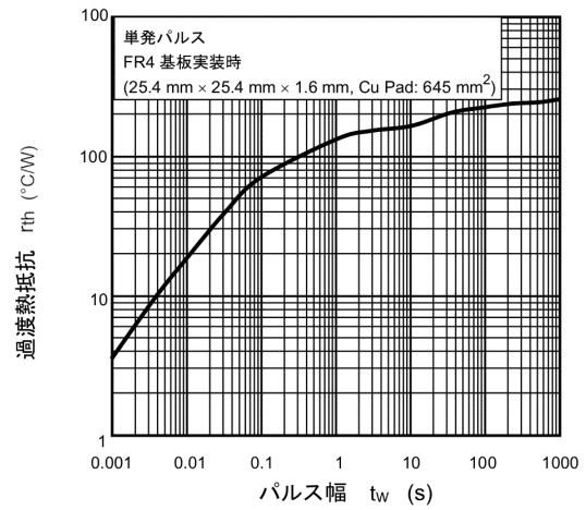
図 7.12 r_{th} - t_w
