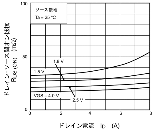
図 7.4 R_{DS(ON)} - I_D
