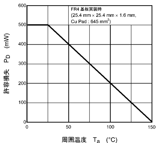
図 7.13 P_D - T_a
