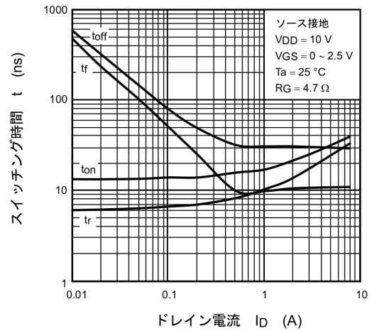
図 7.10 t - I_D
