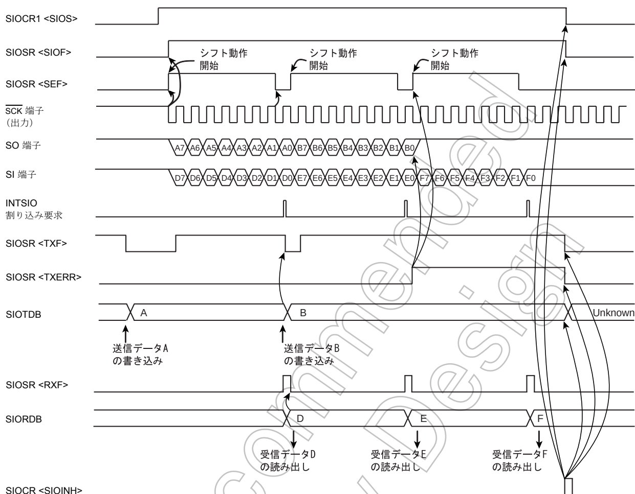
図 11-15 送受信モード (送信) エラー処理の例
