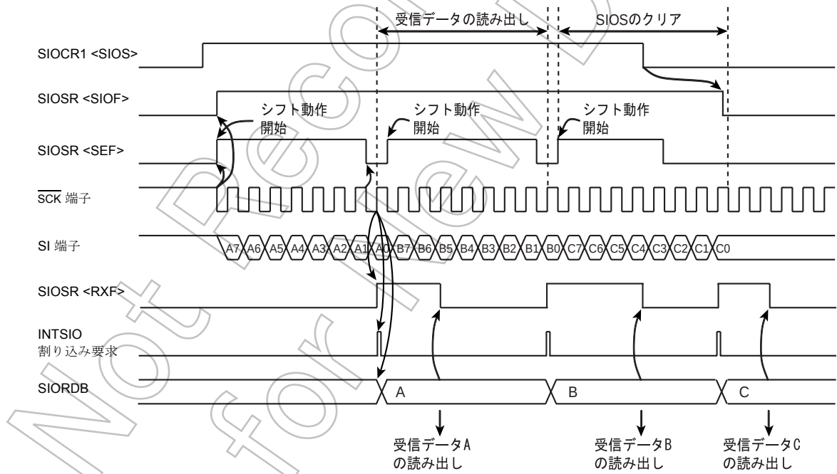
図 11-11 外部クロック、MSB 受信の例
