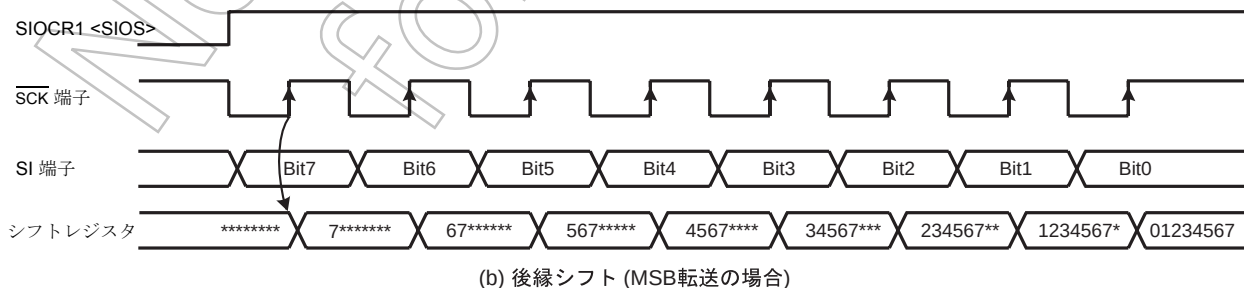
図 11-4 シフトエッジ
