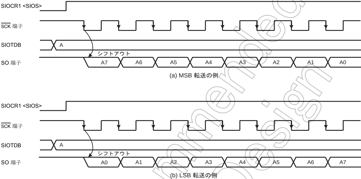
図 11-5 転送ビット方向 ( 送信モードの例 )
