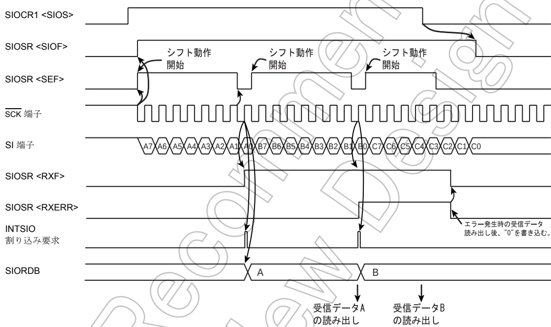
図 11-12 受信モードエラー処理の例
