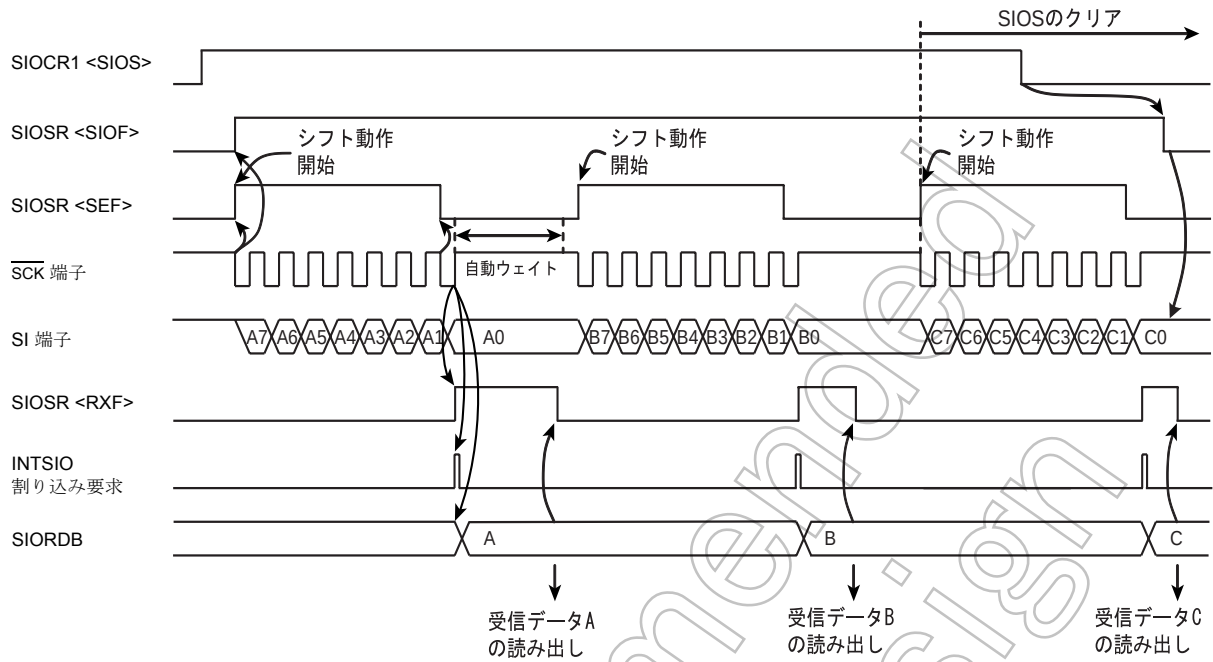
図 11-10 内部クロック、MSB 受信の例
