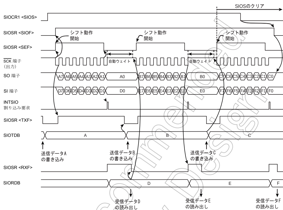
図 11-13 内部クロック、MSB 送受信の例
