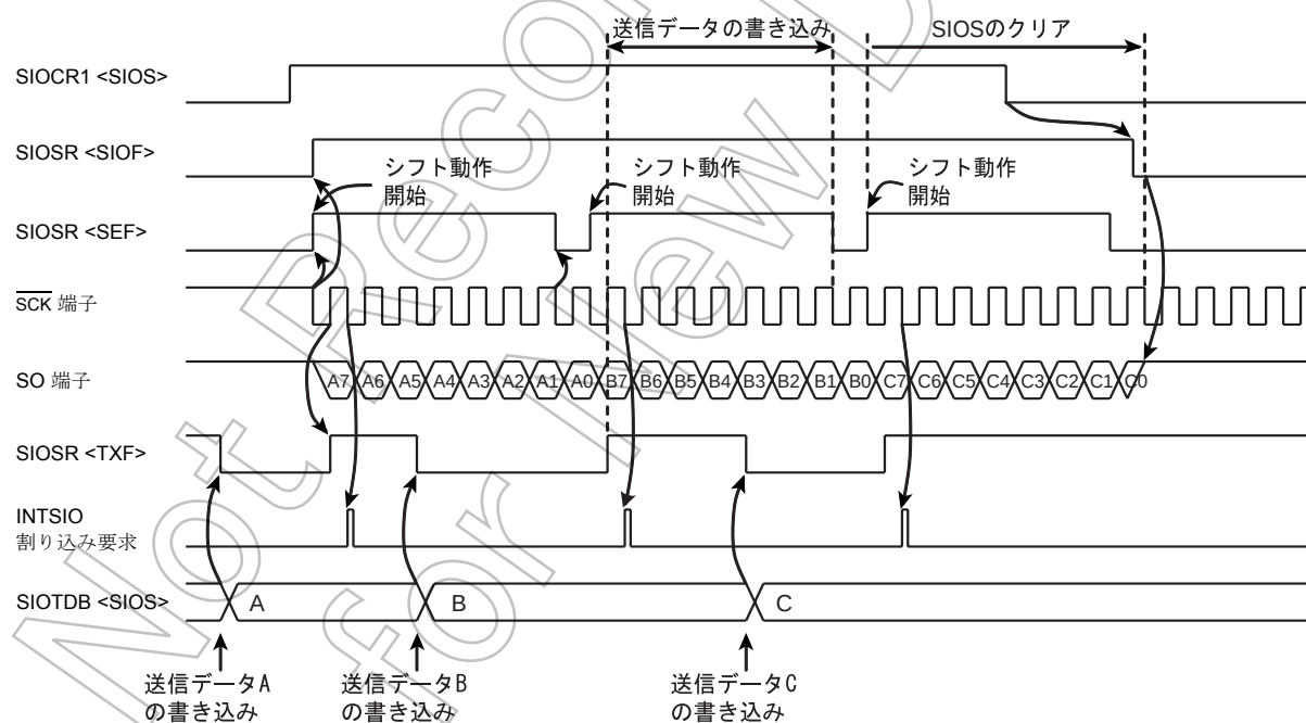
図 11-7 外部クロック、MSB 送信の例
