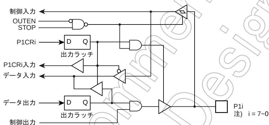
図 5-3 P1 ポート
