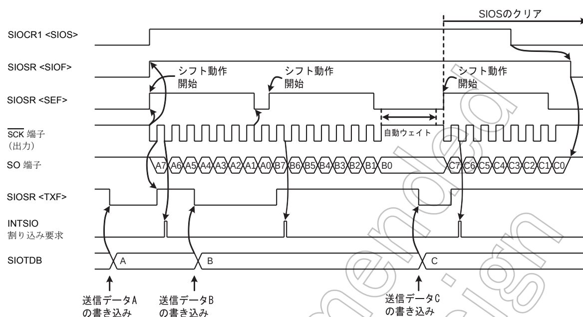
図 11-6 内部クロック、MSB 送信の例
