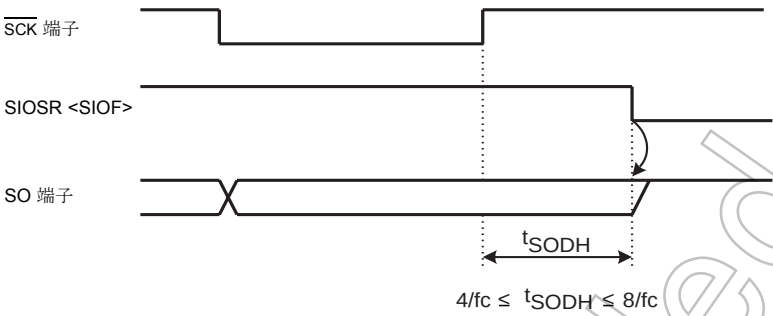
図 11-8 送信終了時のデータ保持時間
