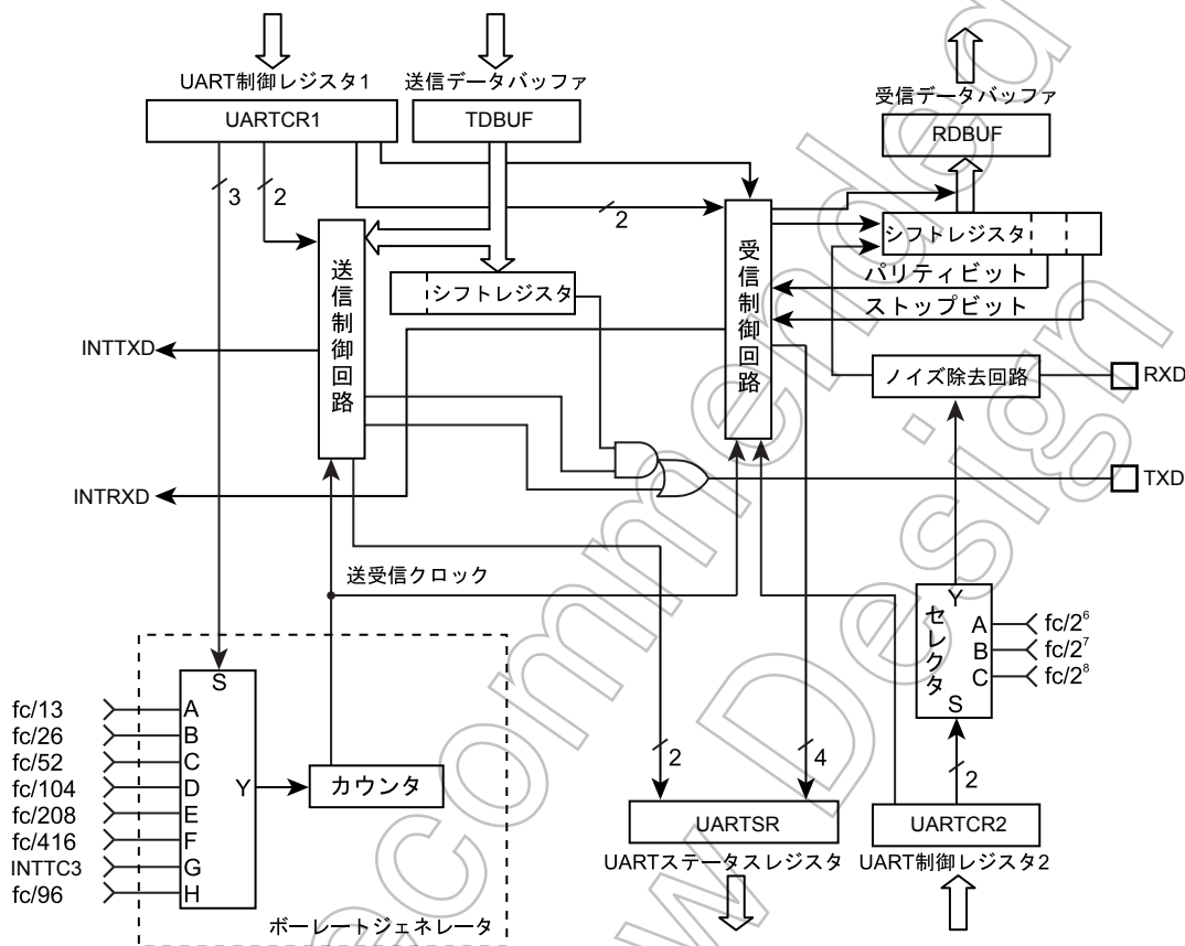
図 12-1 UART ( 非同期型シリアルインタフェース )
