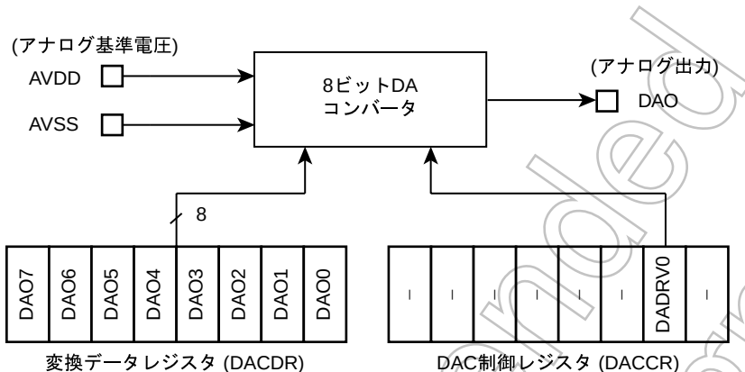
図 14-1 8 ビット DA コンバータ回路構成
