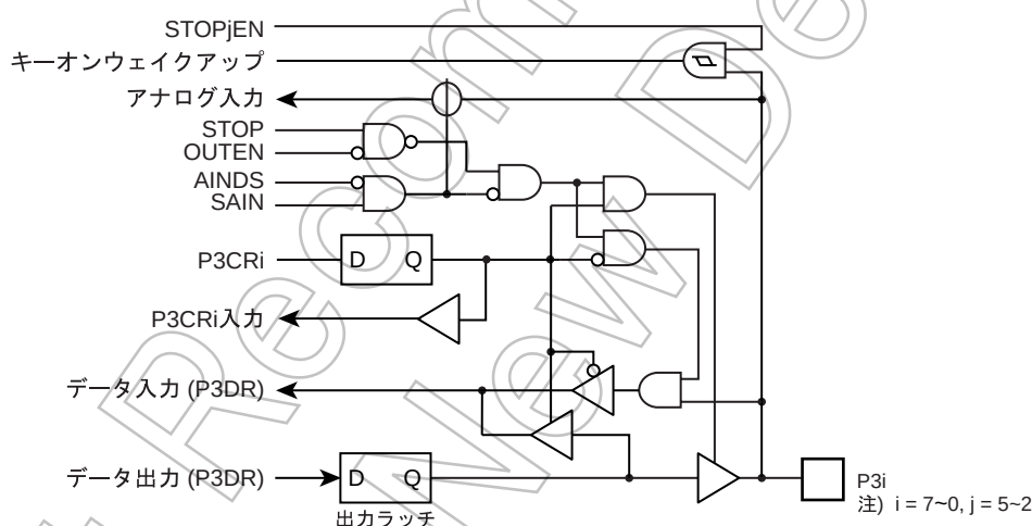
図 5-5 P3 ポート
