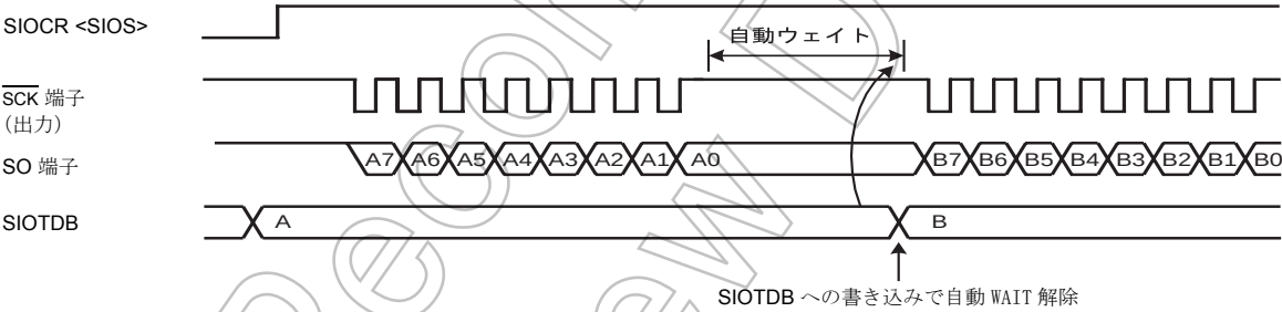
図 11-2 自動ウェイト機能 (送信モードの例)
