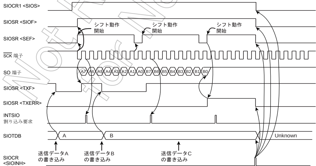
図 11-9 送信モードエラー処理の例
