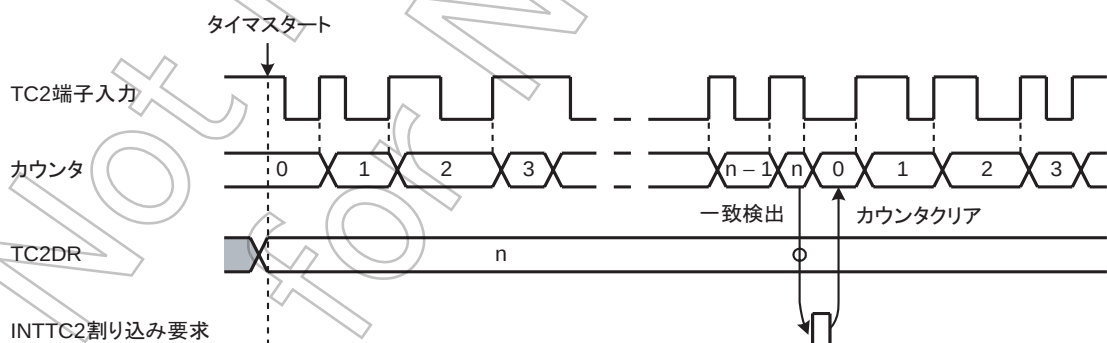
図 9-3 イベントカウンタモードタイミングチャート
