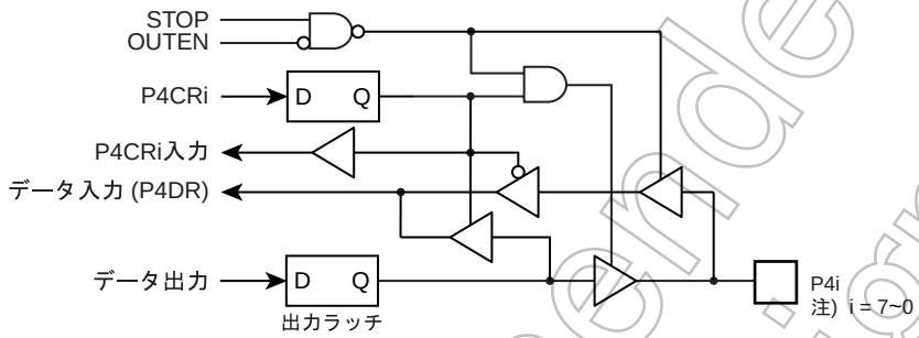
図 5-6 P4 ポート
