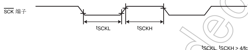
図 11-3 外部クロック
