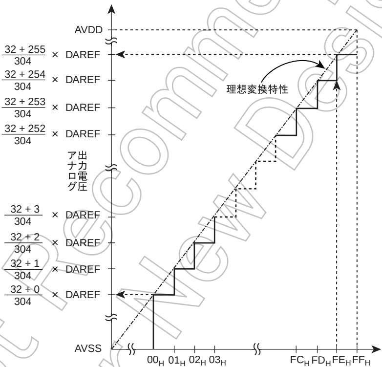
図 14-2 DA 変換値 (8 ビットデジタル入出力コード) と DA 変換されたアナログ出力電圧の関係 (理想値)
