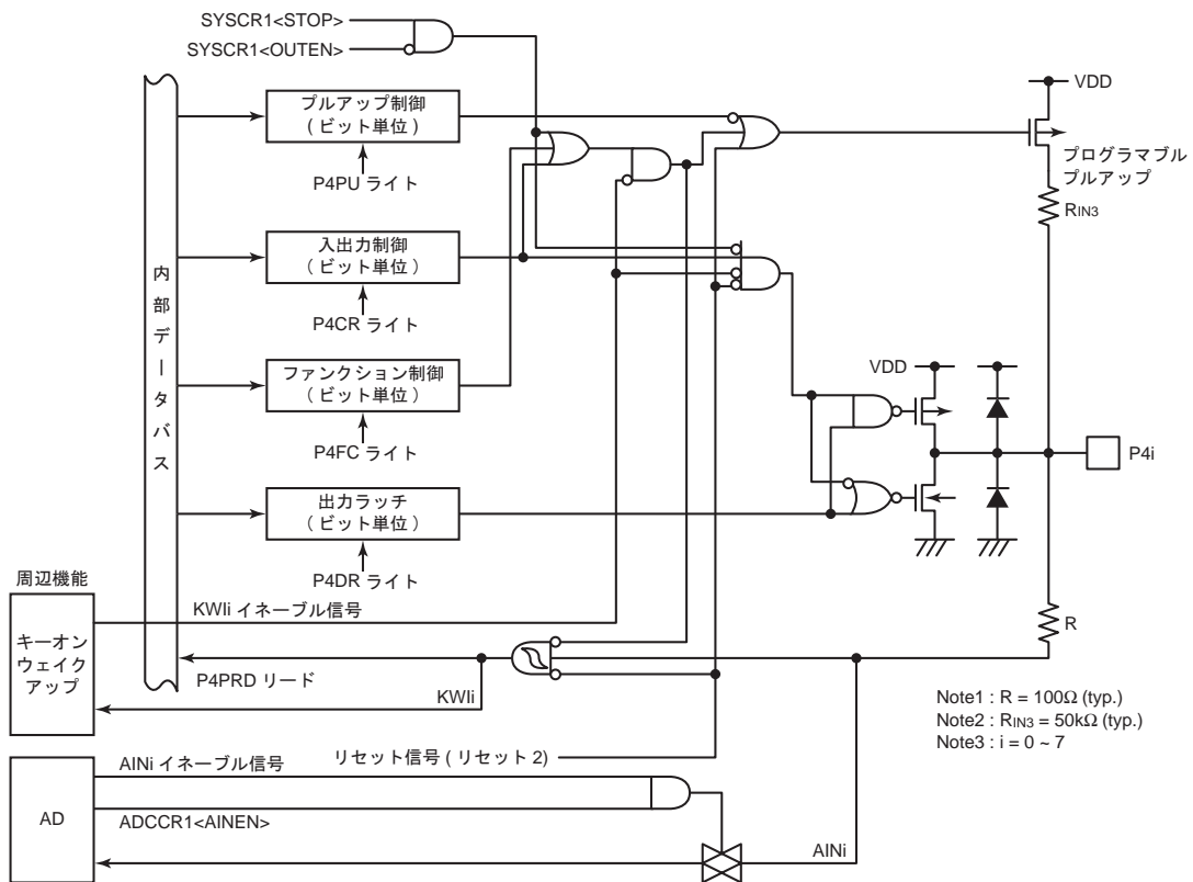
図 8-6 P4 ポート
