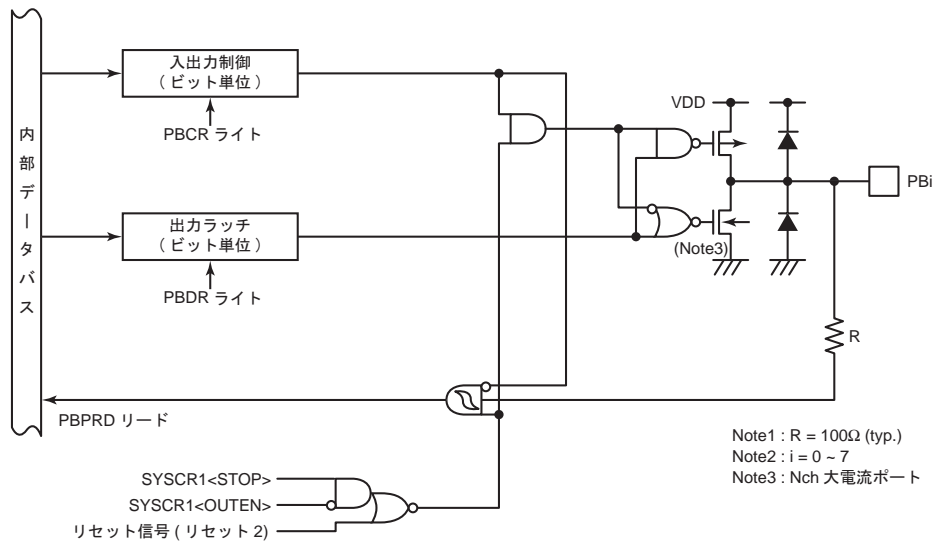
図 8-11 PB ポート
