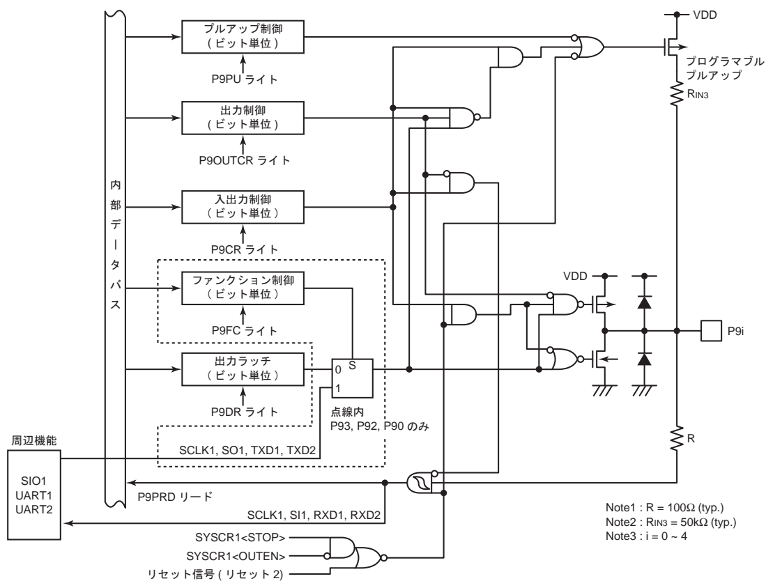
図 8-10 P9 ポート
