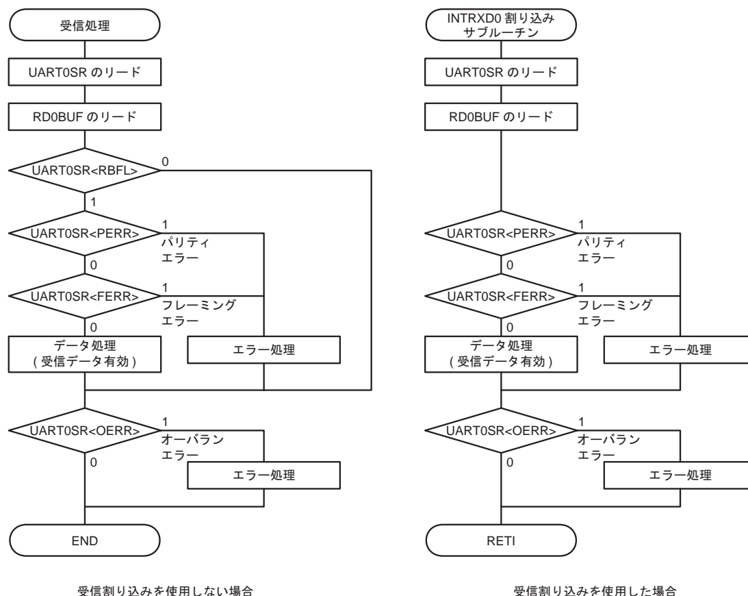
図 16-18 受信処理例
