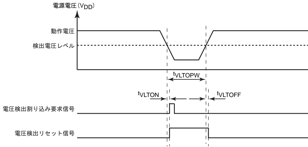
図 25-7 電圧検出回路の動作タイミング
