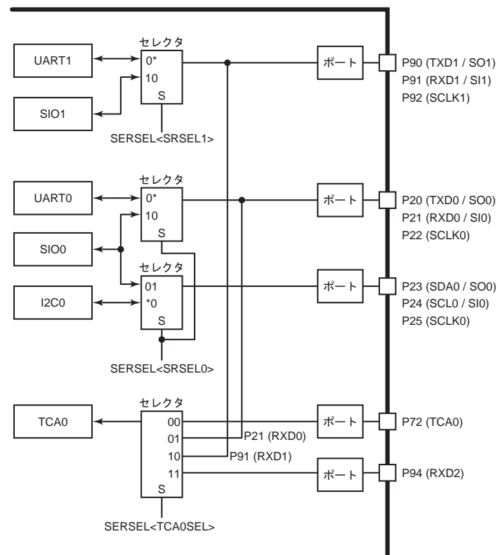
図 8-12 シリアルインタフェース選択機能
