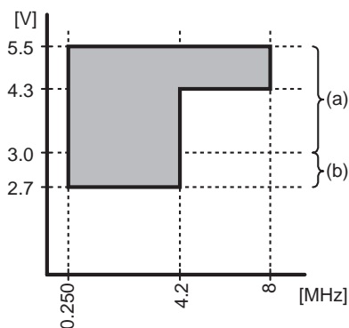
ギアクロック (fcgck) の周波数範囲
