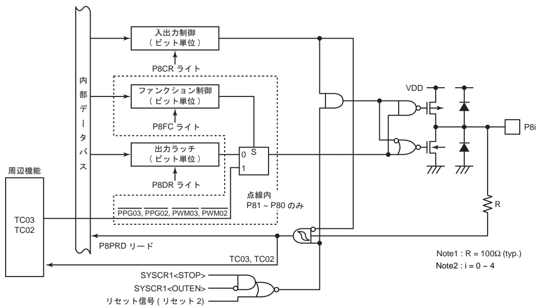
図 8-9 P8 ポート
