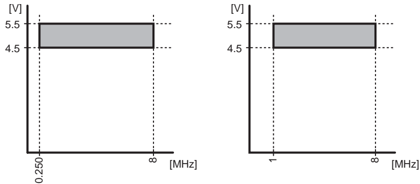
ギアクロック (fcgck) の周波数範囲
