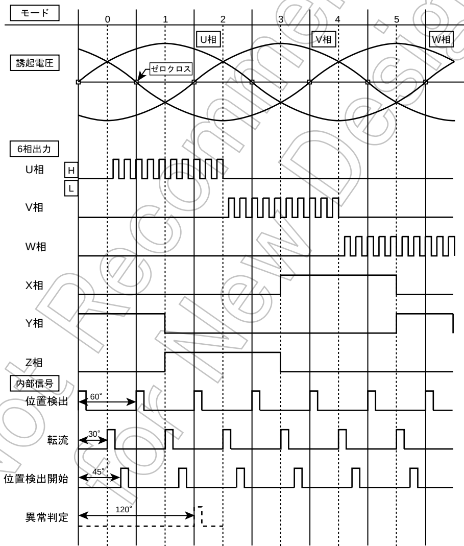
図 13-2 センサレス DC モータの制御タイミングチャート例
