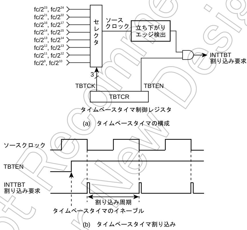
図 6-1 タイムベースタイマ
