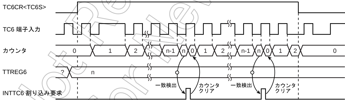
図 12-3 8 ビットイベントカウンタモードタイミングチャート (TC6 の場合)
