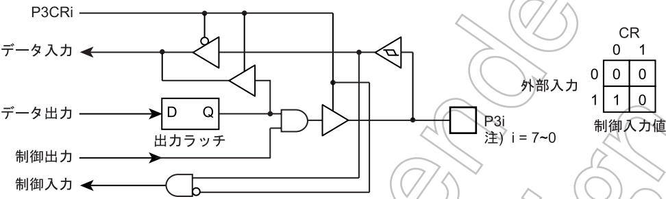
図 5-5 P3 ポート
