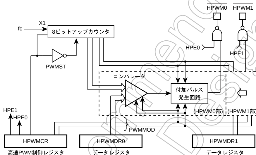
図 17-1 高速 PWM (HPWM0, HPWM1)
