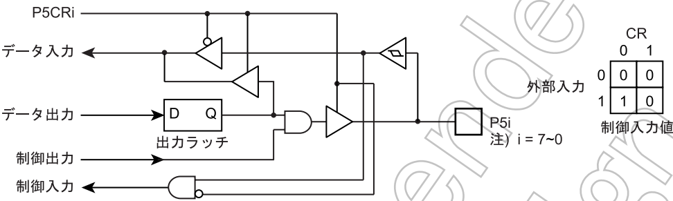
図 5-7 P5 ポート
