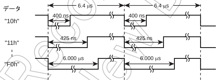
図 17-3 7 ビットモード
