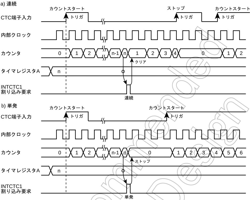
図 9-3 外部トリガモードタイミングチャート
