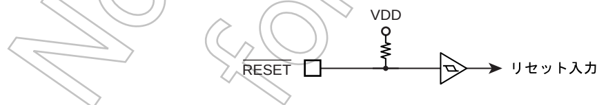
図 2-12 リセット回路
