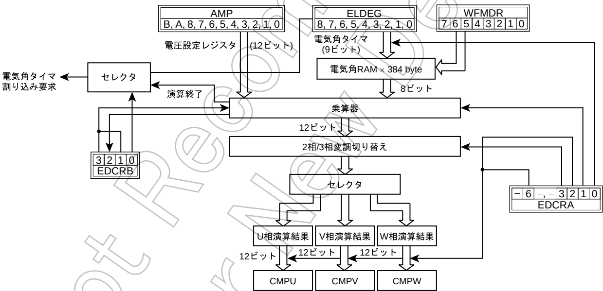
図 13-16 波形演算回路
