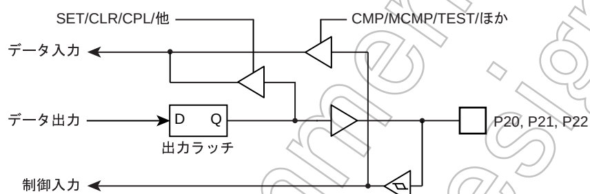
図 5-4 P2 ポート
