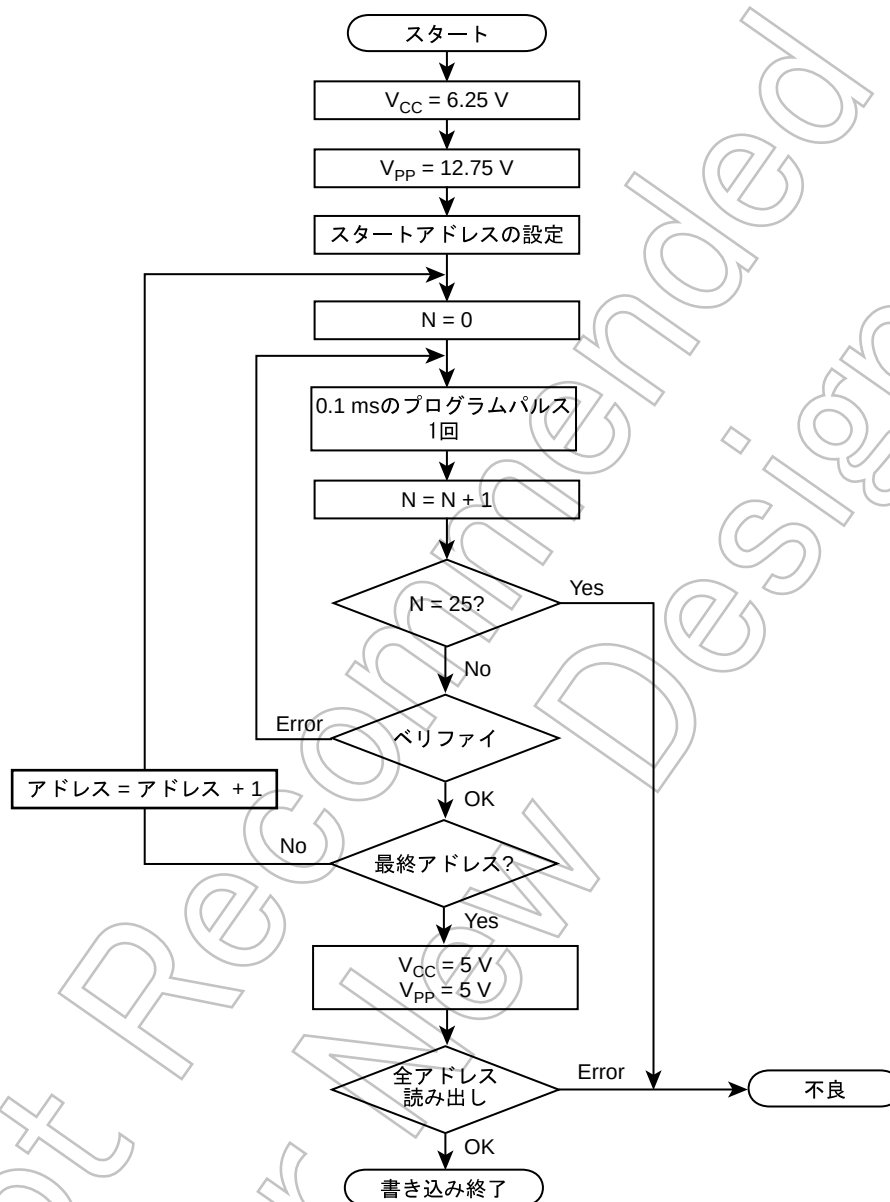
図 18-3 書き込みフローチャート
