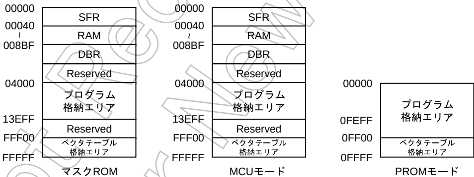
図 18-1 プログラム格納エリア
