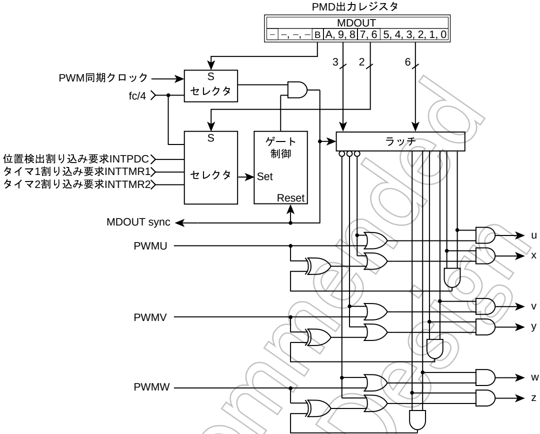
図 13-11 転流制御回路
