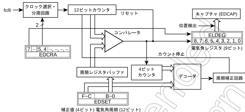
図 13-15 電気角タイマ回路
