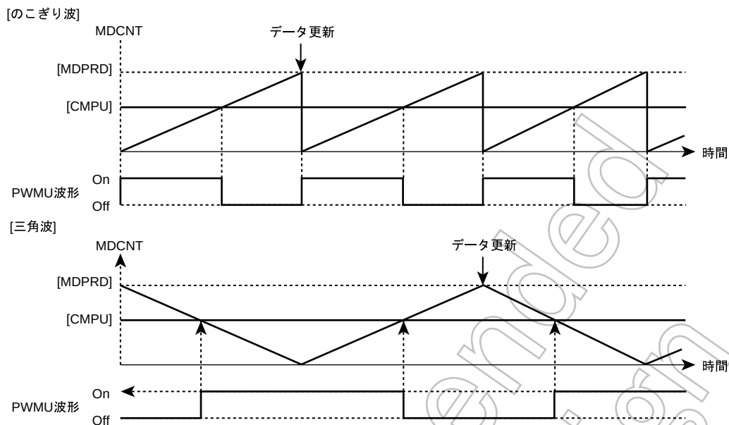
図 12-9 PWM 波形
