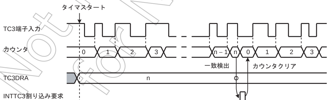
図 10-4 イベントカウンタモードタイミングチャート
