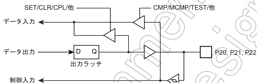
図 5-3 P2 ポート
