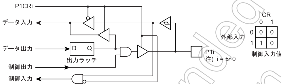
図 5-2 P1 ポート
