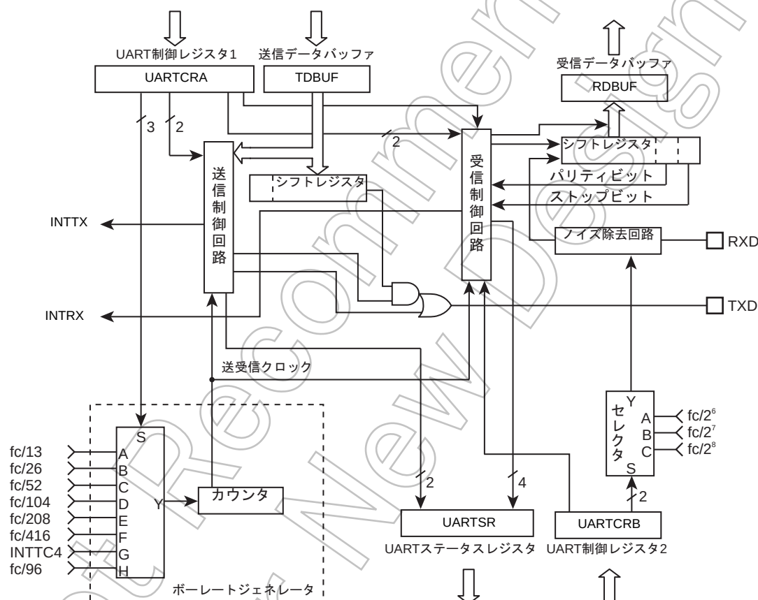
図 13-1 UART (非同期型シリアルインタフェース)
