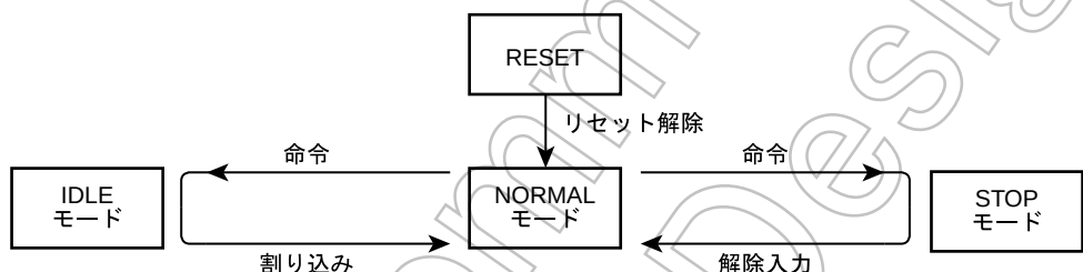
図 2-6 動作モード状態遷移図
