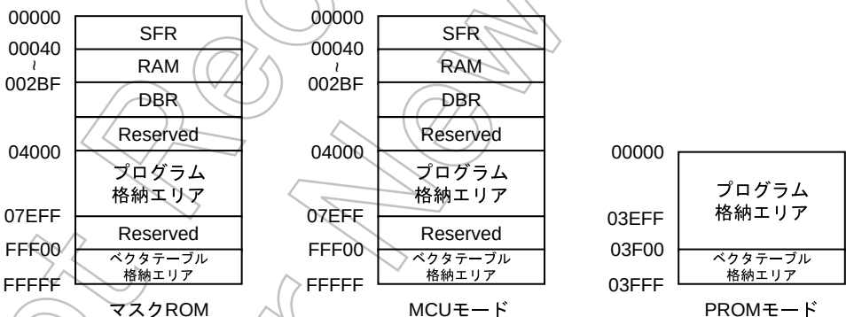
図 16-1 プログラム格納エリア
