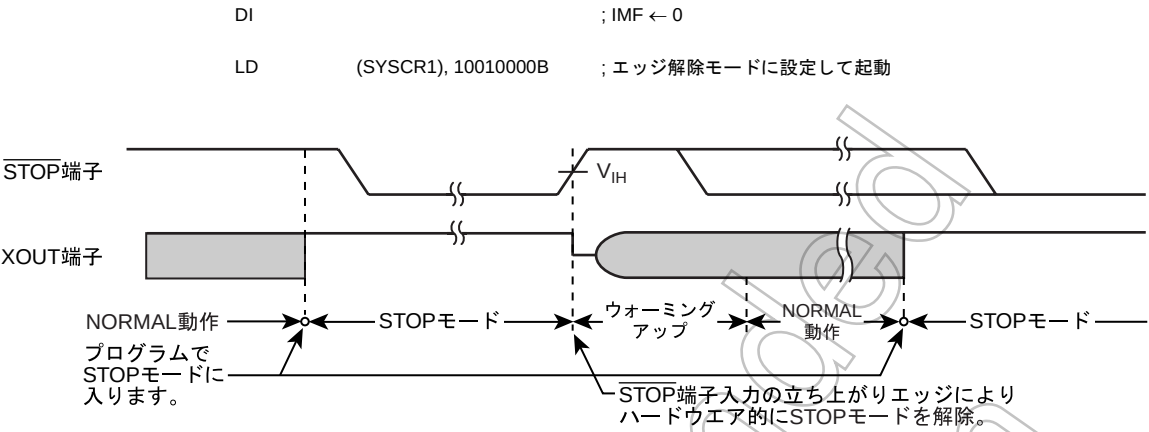
図 2-8 エッジ解除モード
