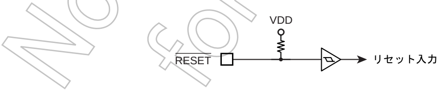
図 2-12 リセット回路
