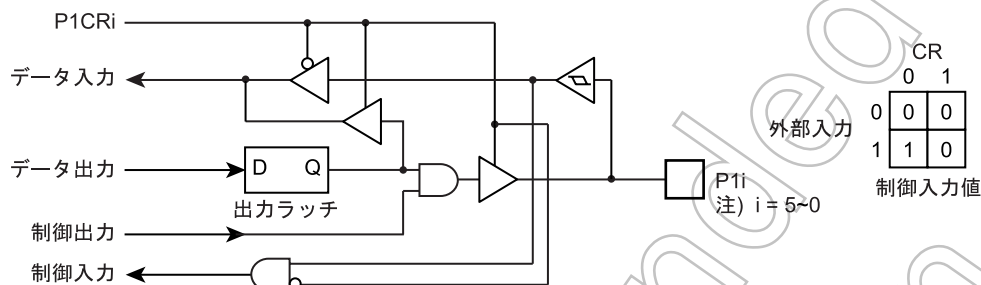
図 5-2 P1 ポート
