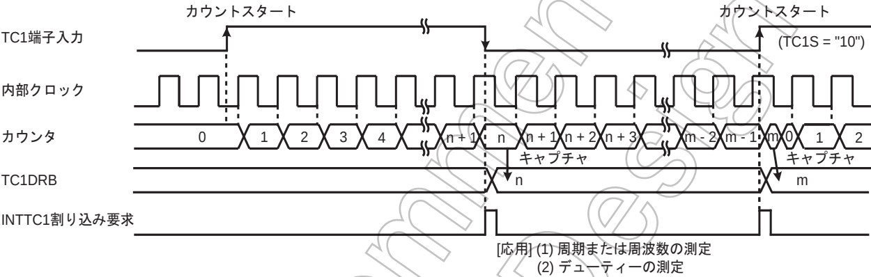
(b) 両エッジキャプチャ (MCAP1 = "0")
