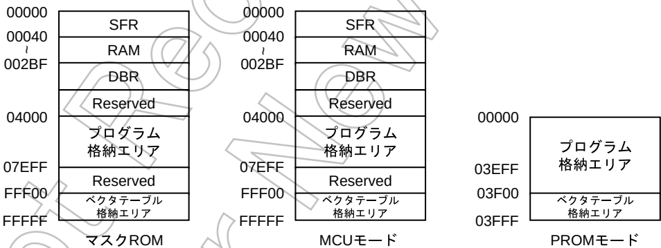
図 16-1 プログラム格納エリア
