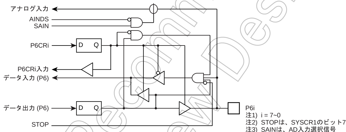
図 5-6 P6 ポート
