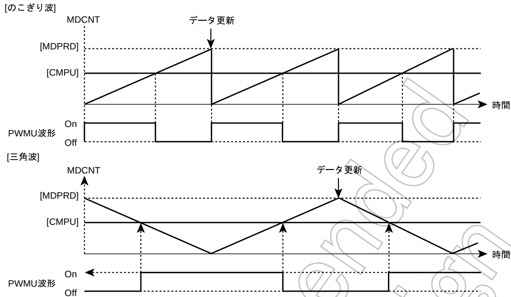
図 12-9 PWM 波形
